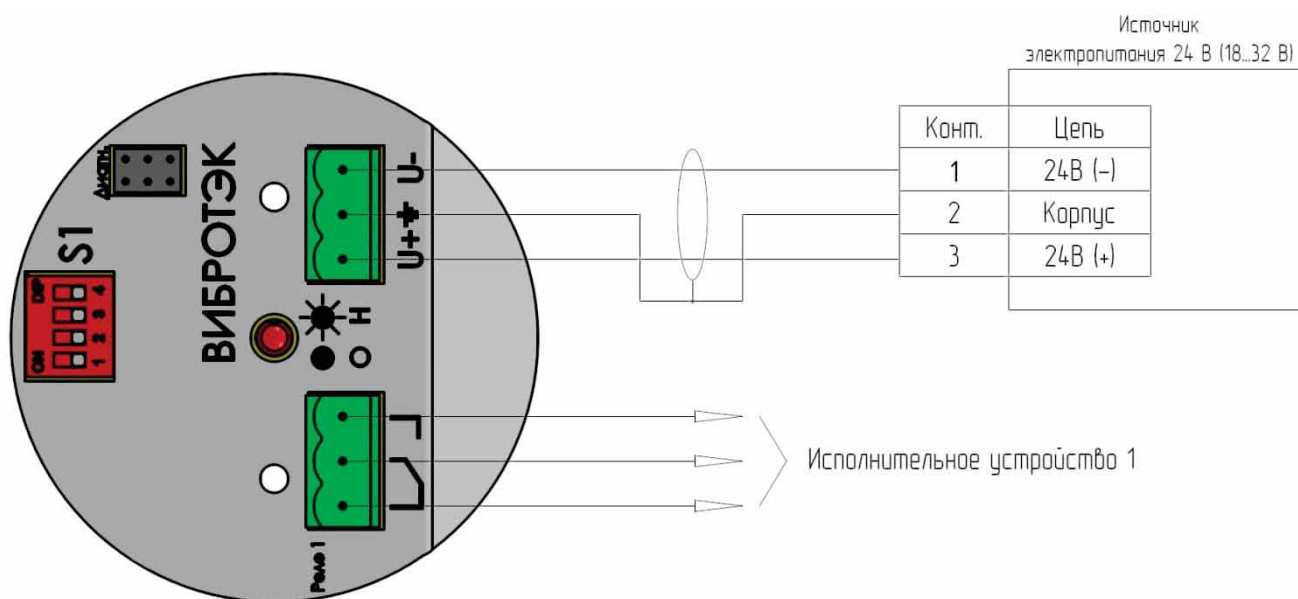
Рисунок 29 – Подключение сигнализатора исполнения P1 (24 В)
