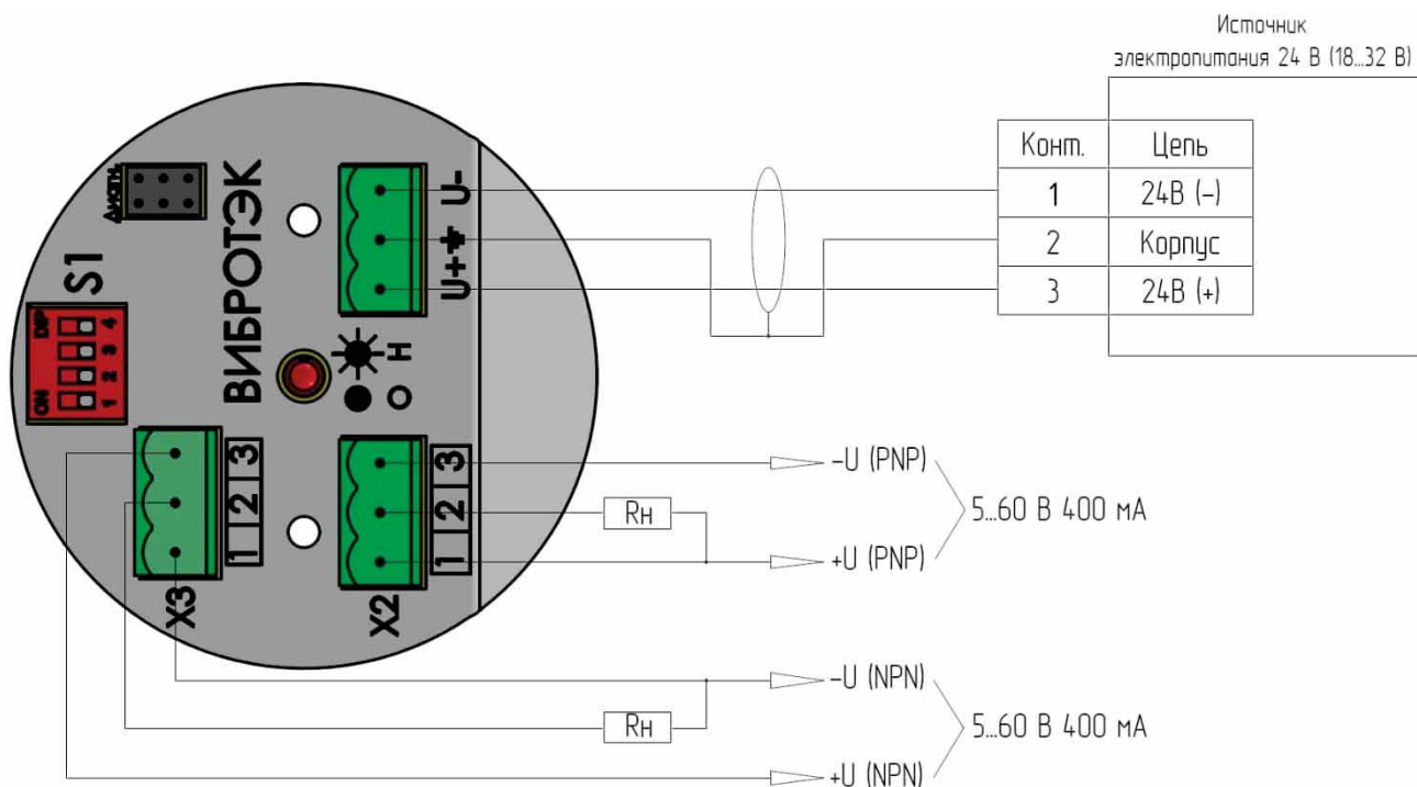
Рисунок 34 – Подключение сигнализатора исполнения ТР5
