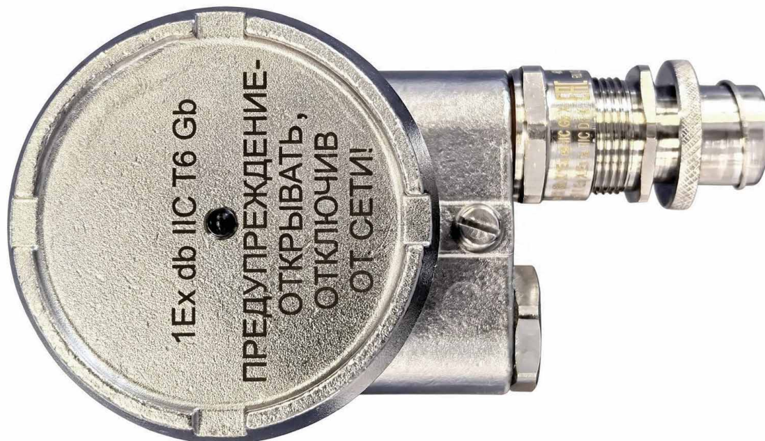
Рисунок 1 – Вид сигнализатора сверху
