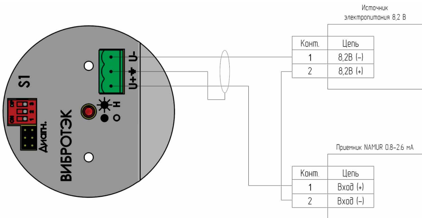
Рисунок 32 – Подключение сигнализатора исполнения Namur
