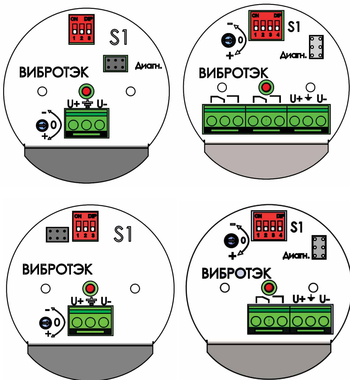
Рисунок 65 – Дискретный регулятор в блоке электронном
