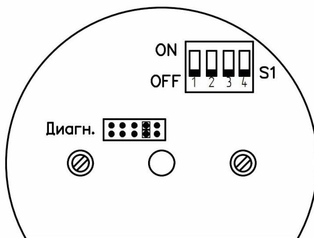
Рисунок 48 – Положение перемычки при переключении сигнализаторов в режим «Диагностика»
