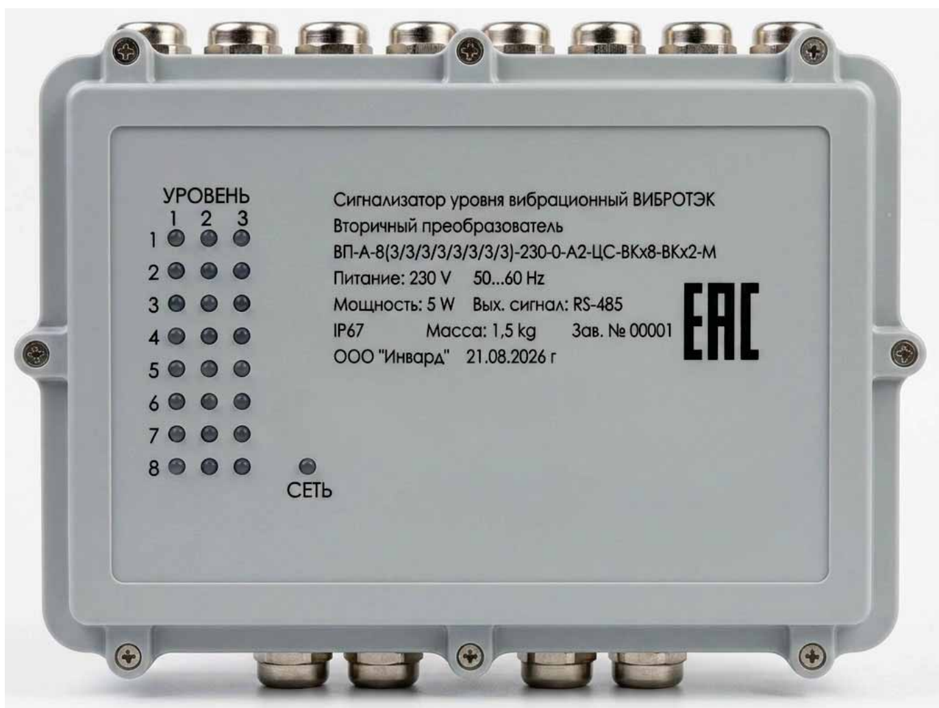
Рисунок 19 – Вторичный преобразователь в алюминиевом корпусе IP54/IP65 для 8 сигнализаторов
