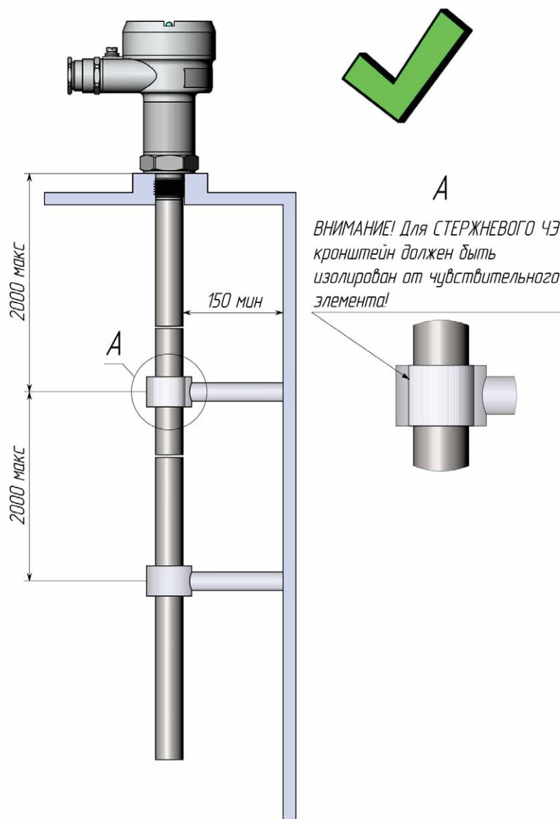
Рисунок 61 – Опоры, необходимые для удлиненного чувствительного элемента
