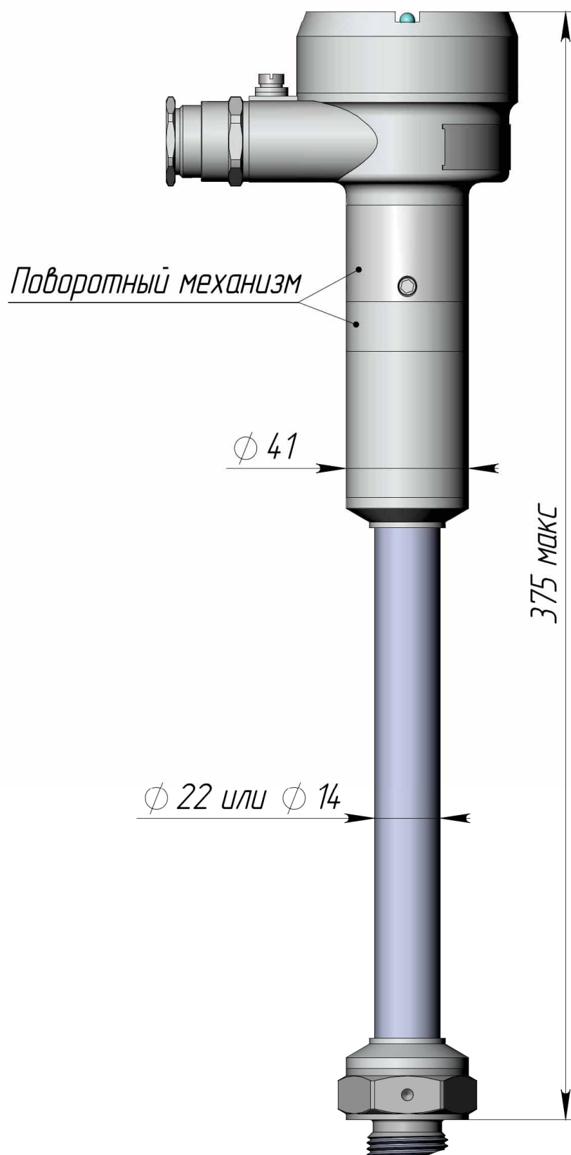
Рисунок В.16 – Габаритные размеры перехода на 450°С с поворотным механизмом
