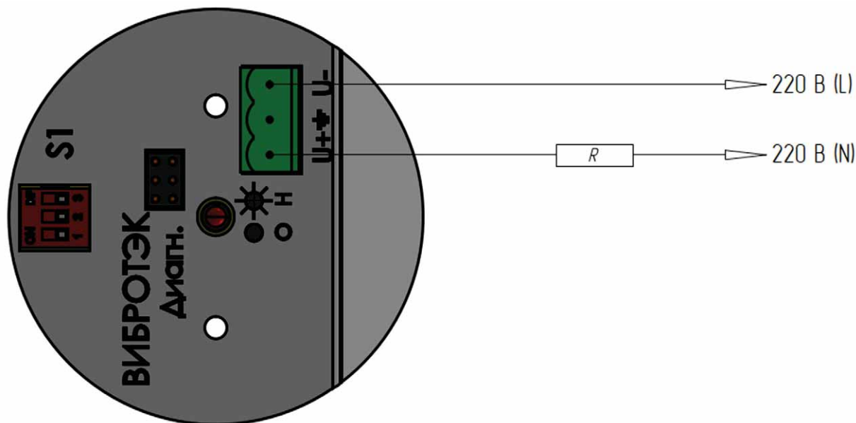
Рисунок 38 – Подключение сигнализатора исполнения БК (220 В)
