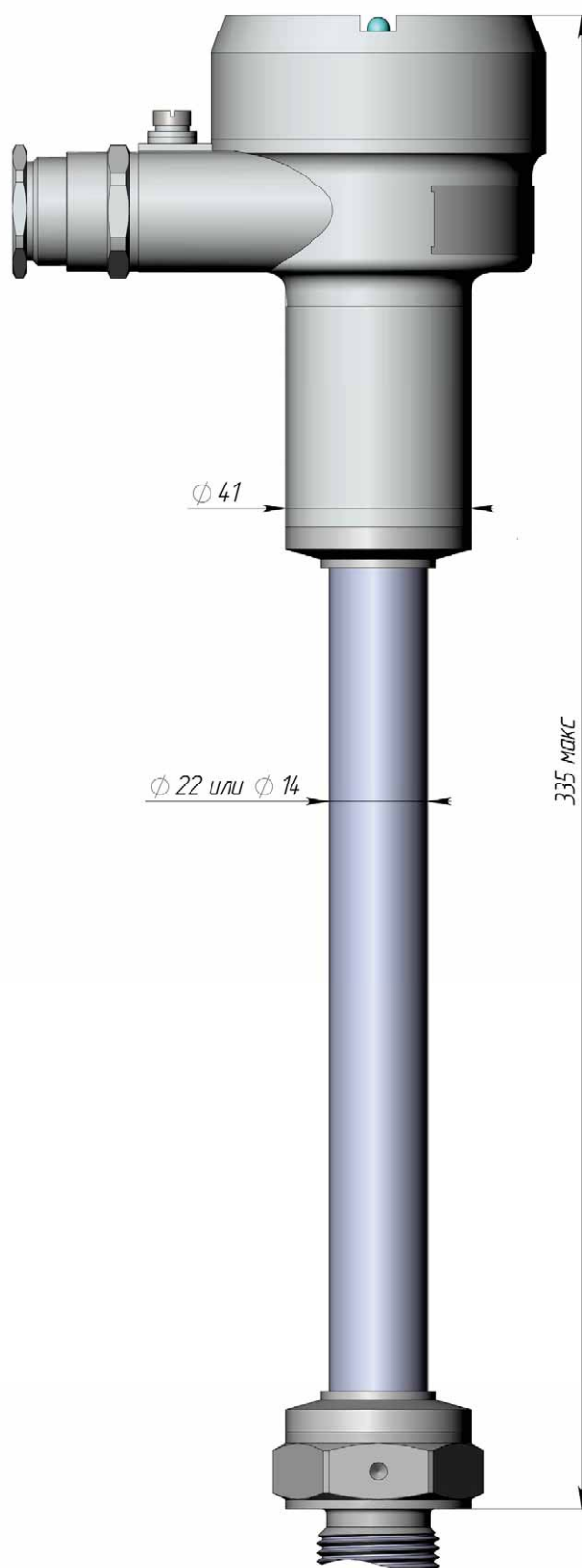
Рисунок В.13 – Габаритные размеры перехода на 450°С
