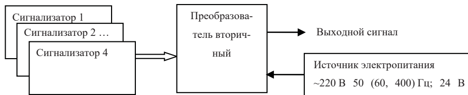
Рисунок 4 – Структурная схема сигнализаторов с вторичным преобразователем
