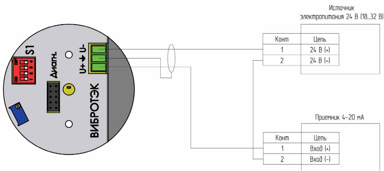
Рисунок 44 – Схема подключения специального исполнения B450 и для сыпучей среды (A1, A2, A3, A4)
