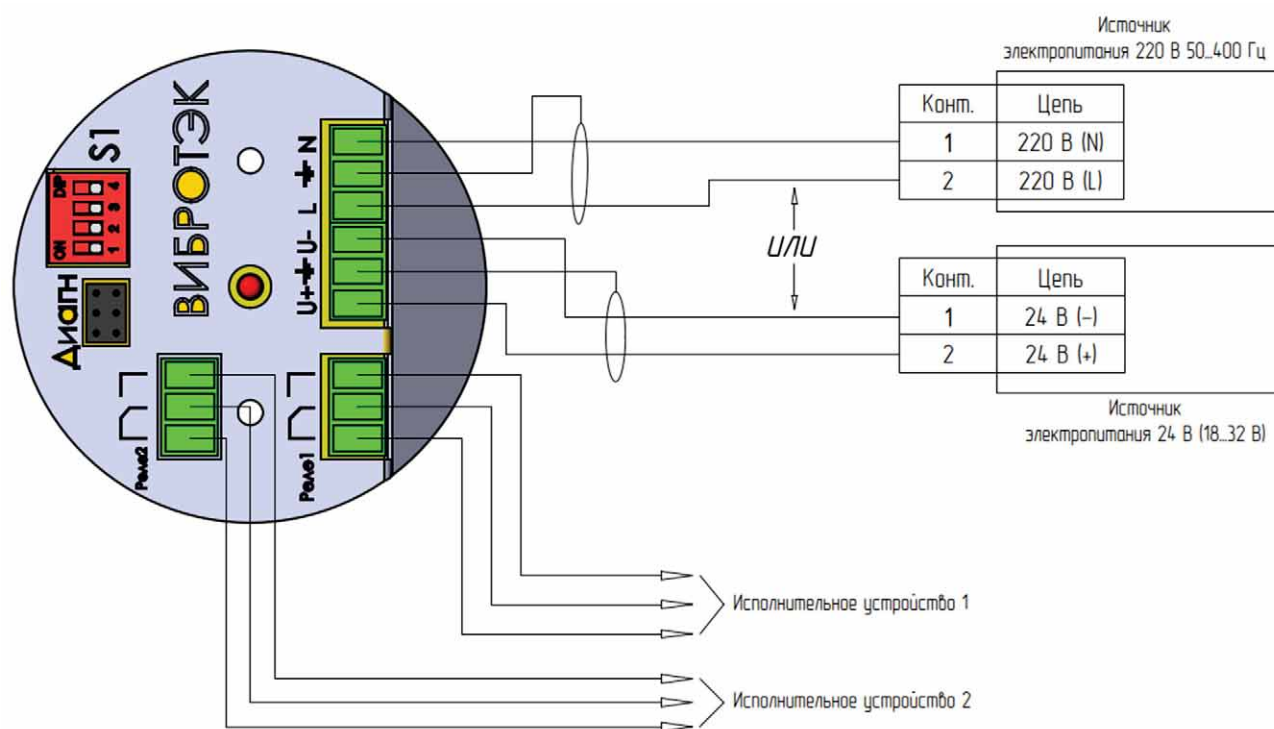
Рисунок 35 – Подключение сигнализатора исполнения Р2, РД, РР (220 В/24В)
