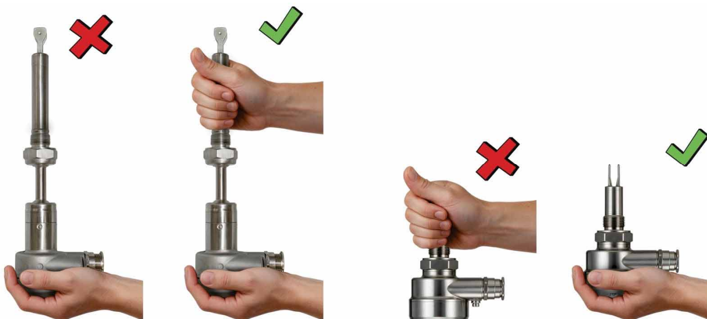
Рисунок 59 – Обращение с сигнализатором
