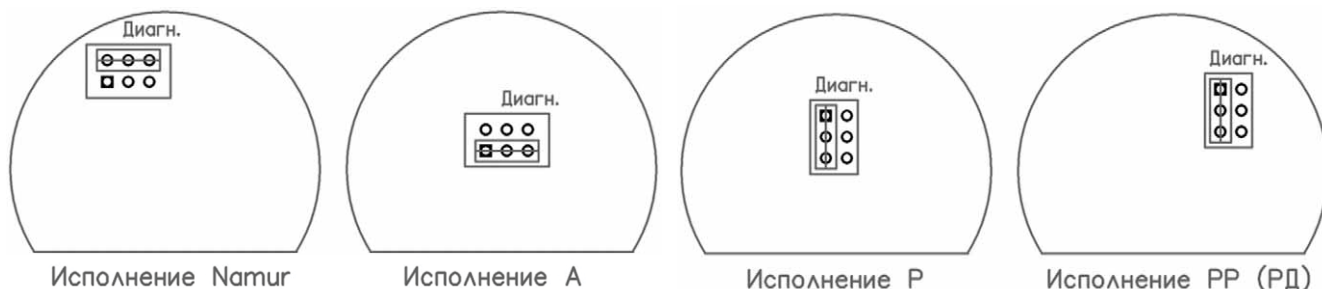
Рисунок 49 – Положение перемычки при переключении сигнализаторов в режим «Настройка порога»
