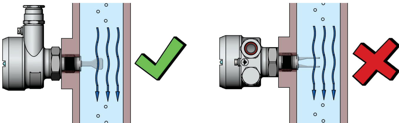
Рисунок 62 – Установка сигнализаторов в трубопроводе
