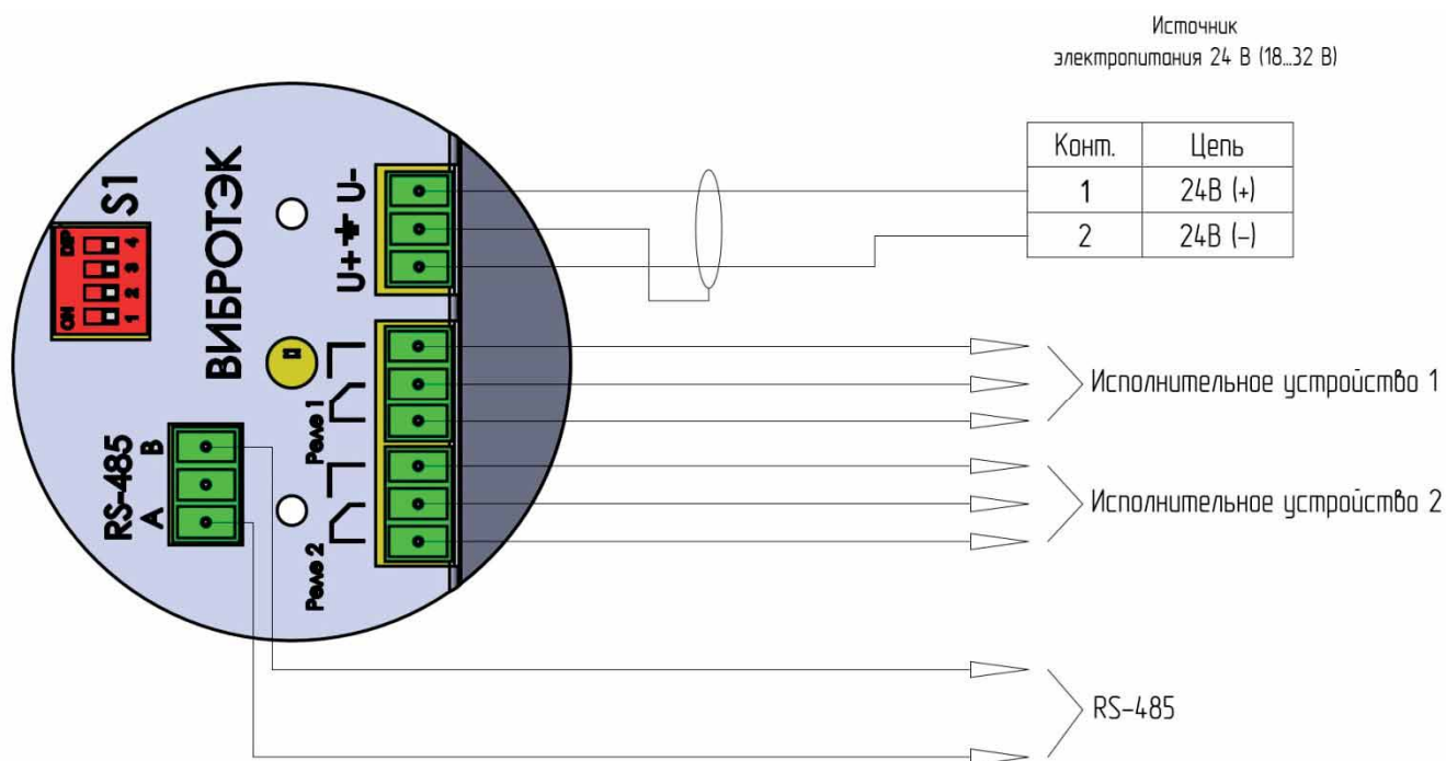
Рисунок 39 – Подключение сигнализатора исполнения БК (24 В)
