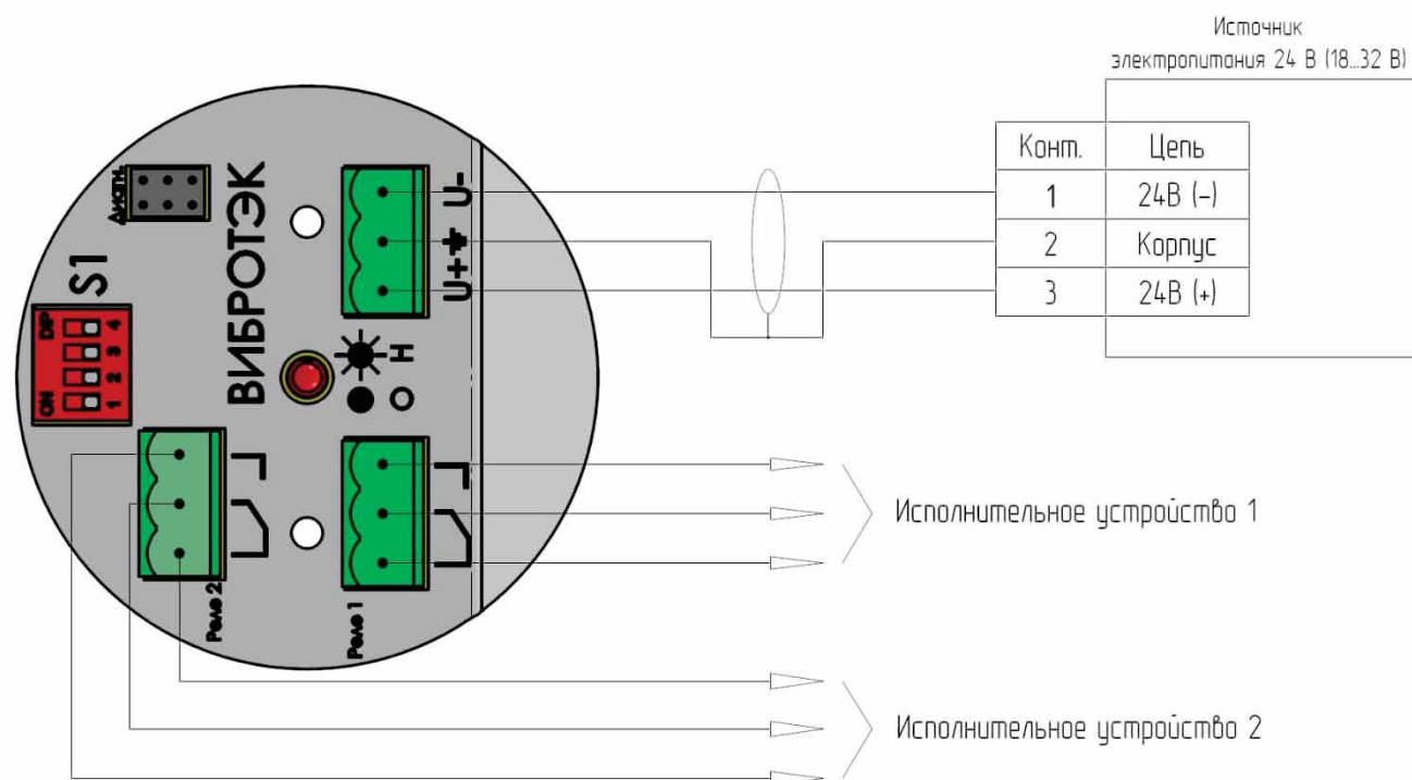
Рисунок 30 – Подключение сигнализатора исполнения P2, PД, PР (24 В)
