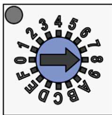
Рисунок 66 – Дискретный регулятор
