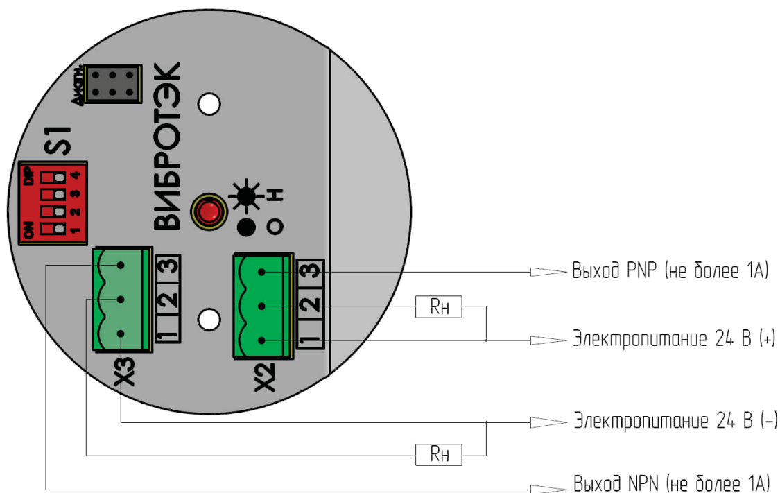
Рисунок 33 – Подключение сигнализатора исполнения ТР3
