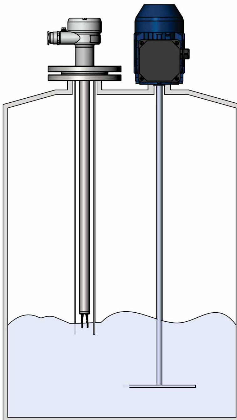
Рисунок 63 – Установка сигнализатора в успокоительной трубе
