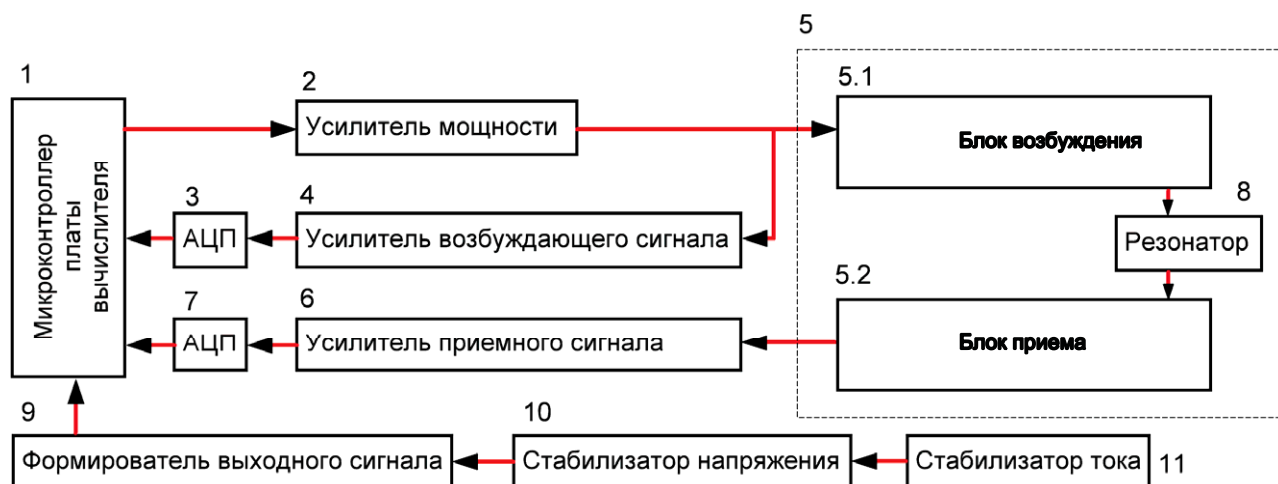
Рисунок 3 – Структурная схема сигнализаторов
