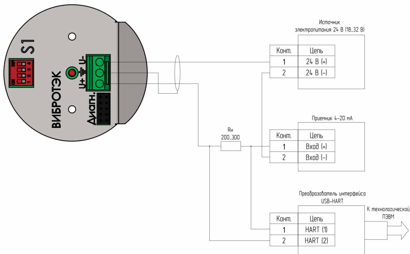
Рисунок 41 – Подключение сигнализатора исполнения А2Н, А3Н
