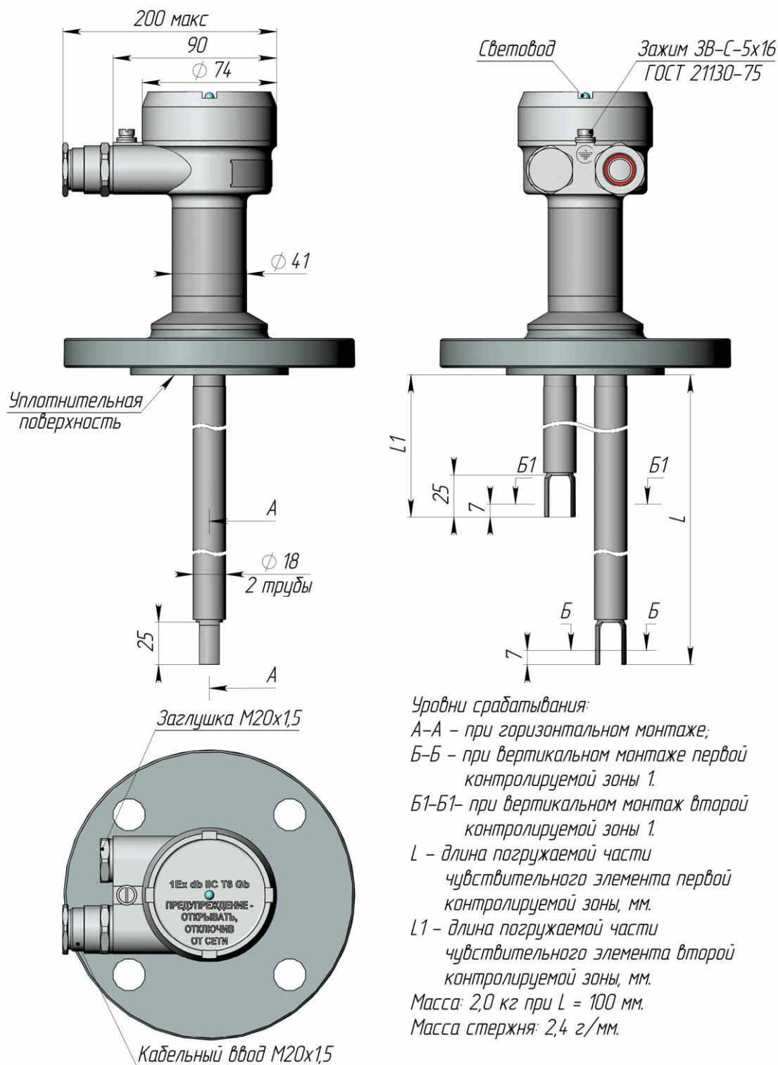
Рисунок В.42 – Габаритные и установочные размеры сигнализатора уровня ВИБРОТЭК-У-М-В с двумя точками контроля. Способ присоединения – фланец, температура контролируемой среды не более 160 °С.
