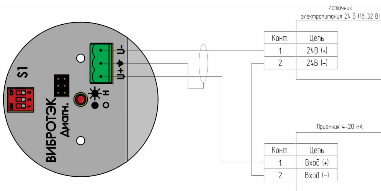
Рисунок 31 – Подключение сигнализатора исполнения A1, A2, A3
