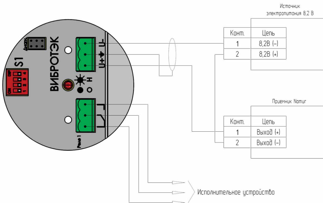
Рисунок 37 – Подключение сигнализатора исполнения Namur / P
