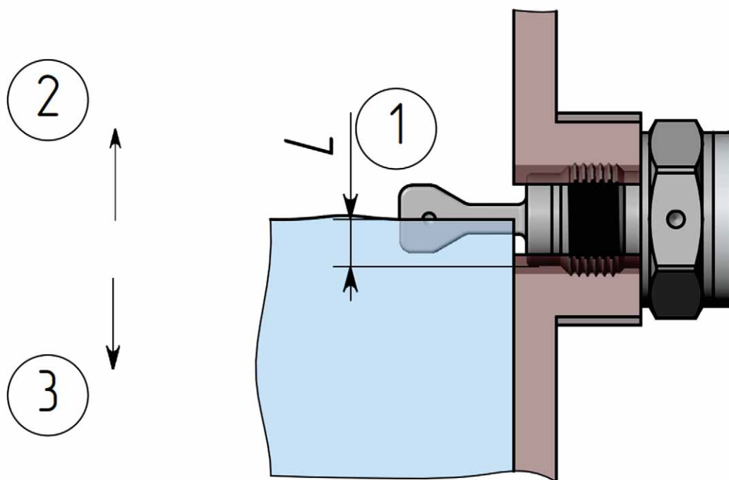
Рисунок 57 – Горизонтальный монтаж
