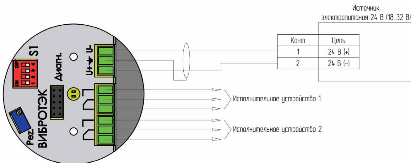
Рисунок 47 – Схема подключения специального исполнения В450 и для сыпучей среды (РД, РР (РА))
