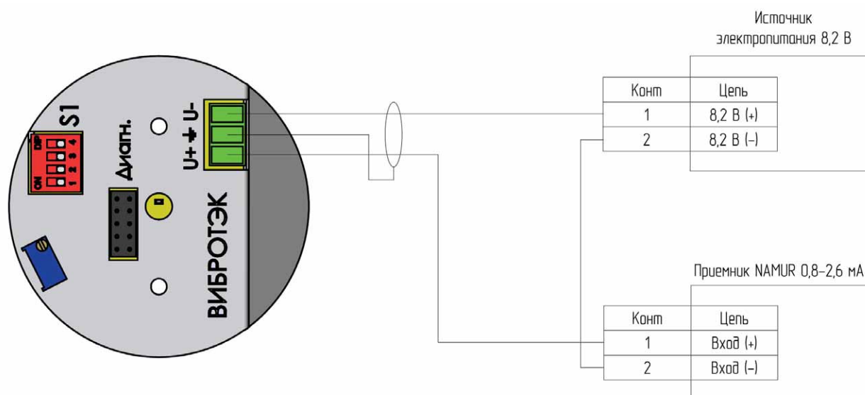
Рисунок 45 – Схема подключения специального исполнения B450 и для сыпучей среды (Namur)
