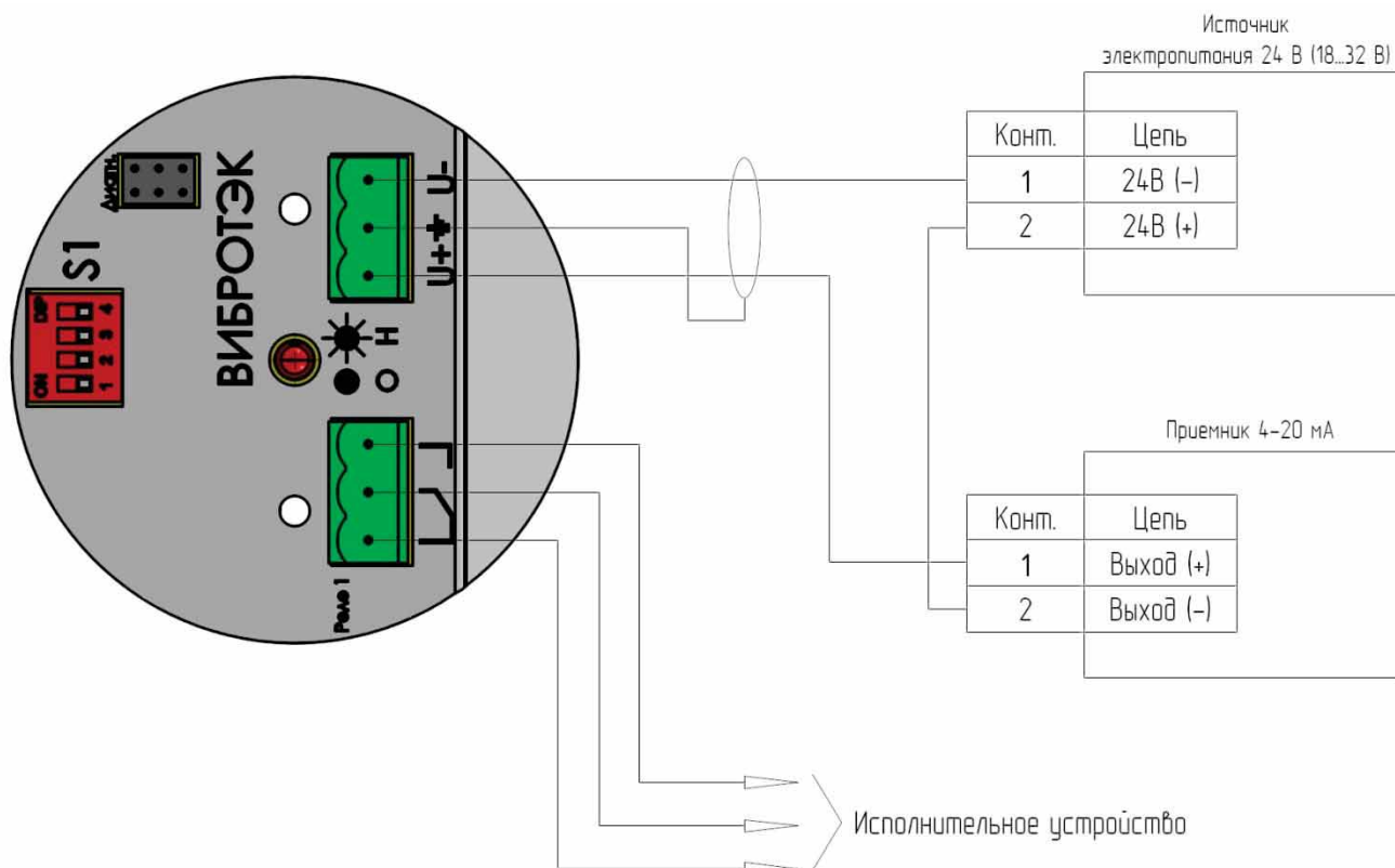
Рисунок 35 – Подключение сигнализатора исполнения Р2, РД, РР (220 В/24В)
