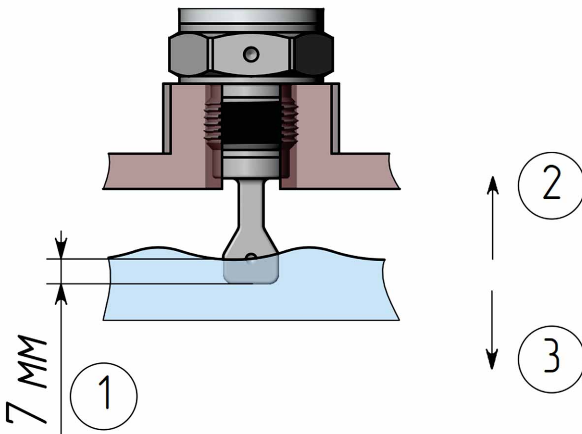
Рисунок 56 – Вертикальный монтаж
