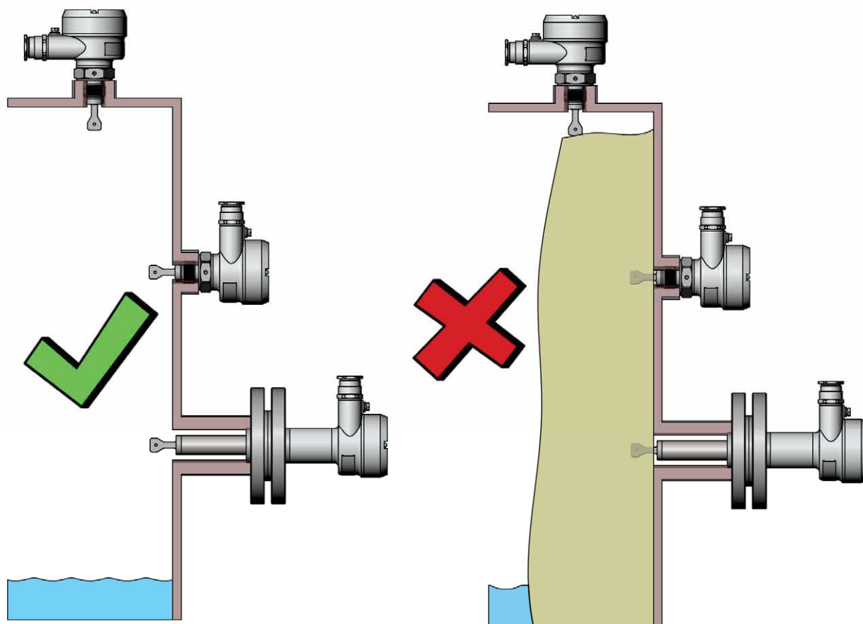
Рисунок 55 – Не допускать образования отложений продукта
