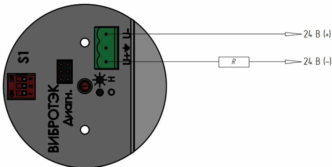
Рисунок 39 – Подключение сигнализатора исполнения БК (24 В)
