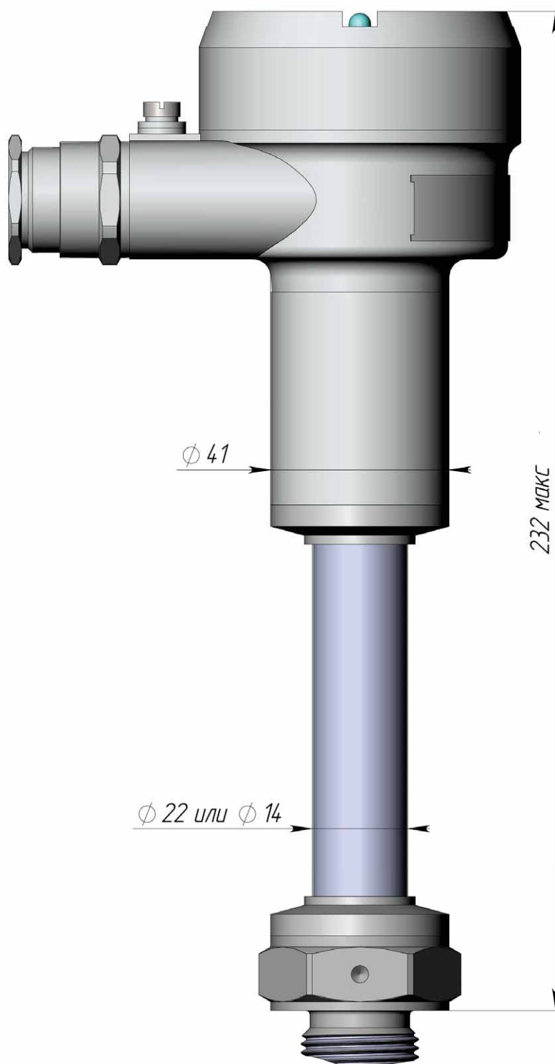
Рисунок В.12 – Габаритные размеры перехода на 250°С
