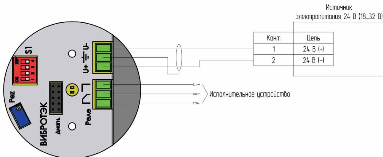
Рисунок 46 – Схема подключения специального исполнения В450 и для сыпучей среды (P1)
