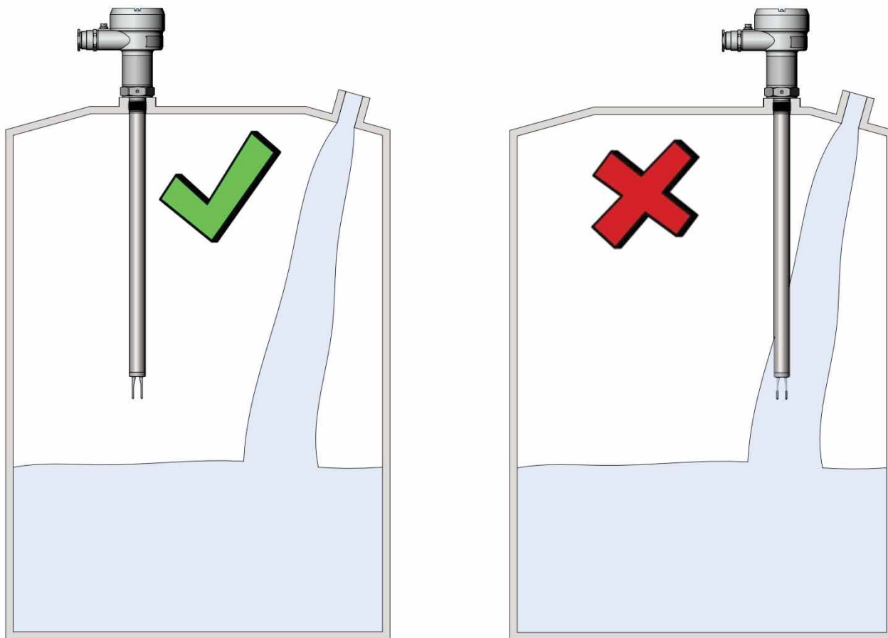
Рисунок 60 – Монтаж сигнализатора относительно трубы налива
