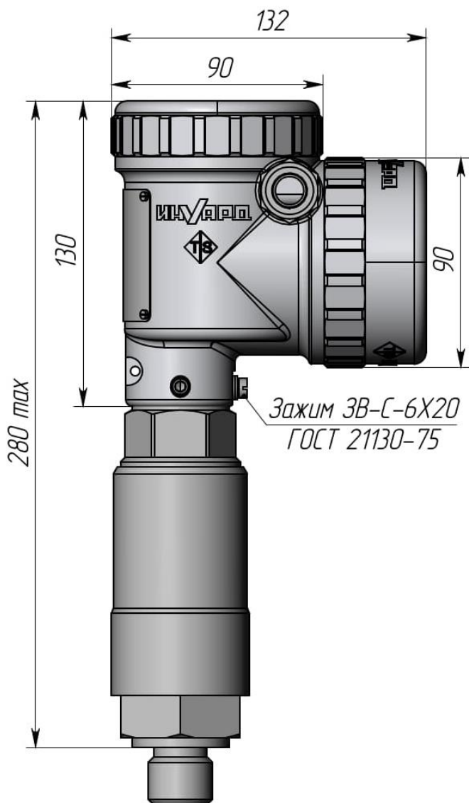
Рисунок Д99 - Габаритные и установочные размеры преобразователей с корпусом мини. Изоляторы ТЕГ. Работа при температуре до 160 °С. Способ присоединения – штуцер. Элемент чувствительный не показан
