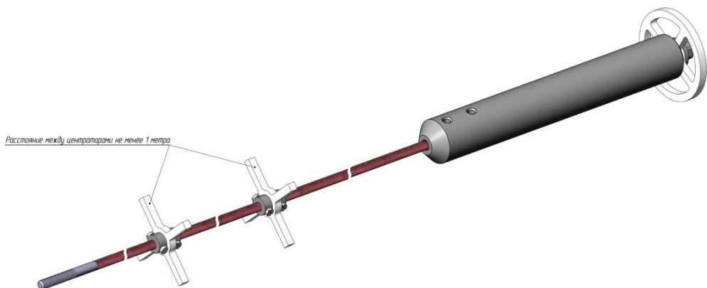
Рисунок E122 – Монтаж керамических центрирующих дисков к одиночному гибкому зонду при помощи нержавеющей втулок для температуры до 500 °С
