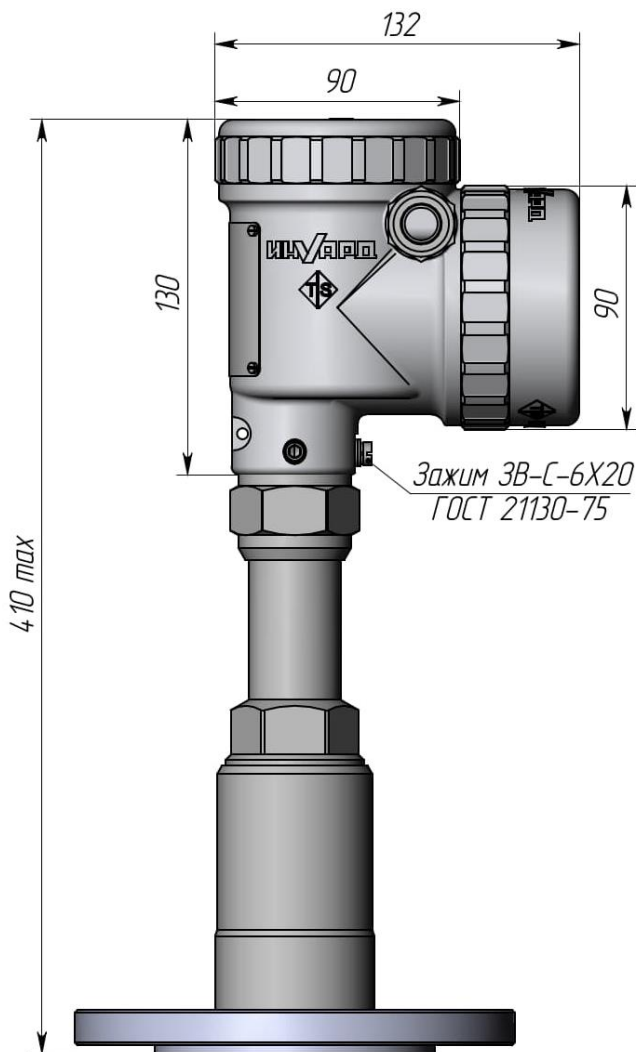
Рисунок Д105 - Габаритные и установочные размеры преобразователей с корпусом мини. Изоляторы ТEG. Работа при температуре до 500 °С. Способ присоединения – фланец. Элемент чувствительный не показан
