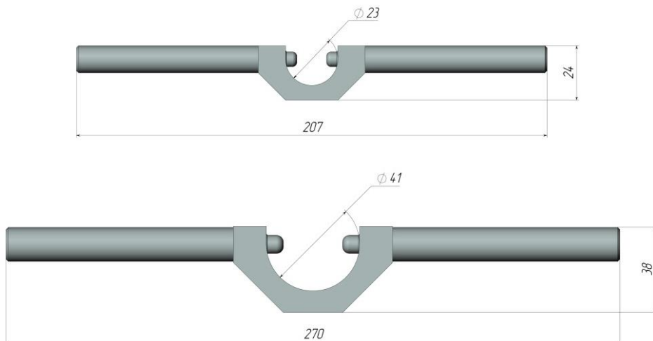
Рисунок М2.1 - Приспособления для сборки (демонтажа)
