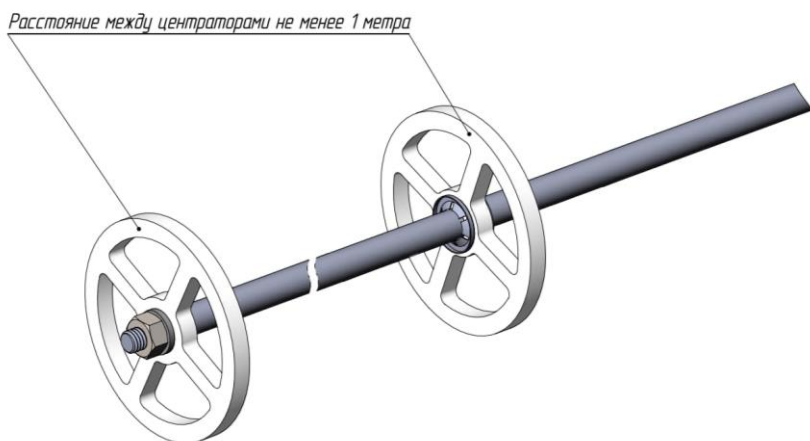
Рисунок Е4 – Монтаж центрирующего диска к одиночным жестким зондам
