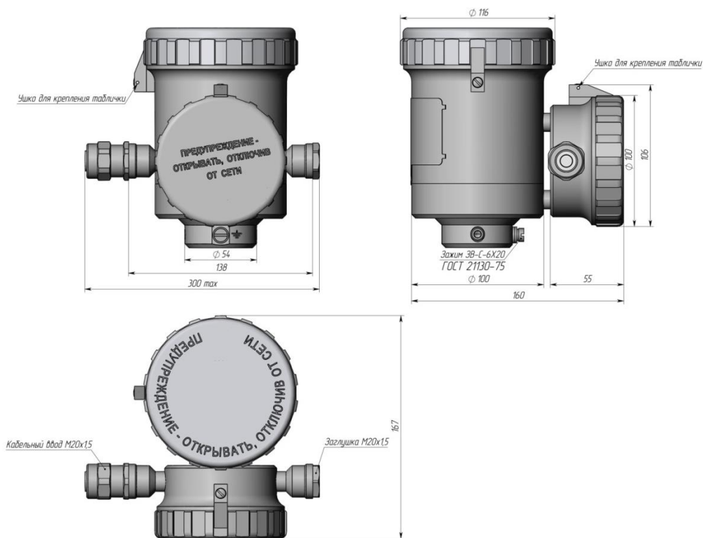
Рисунок Д114 - Габаритные и установочные размеры корпуса из нержавеющей стали блока электронного преобразователя. Класс безопасности ЗН. IP68
