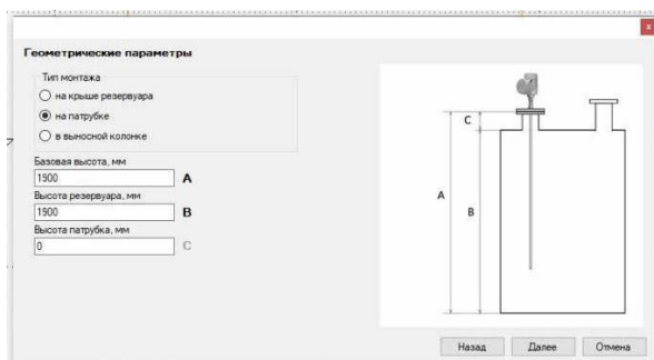
Рисунок 49. Вариант монтажа на трубке
