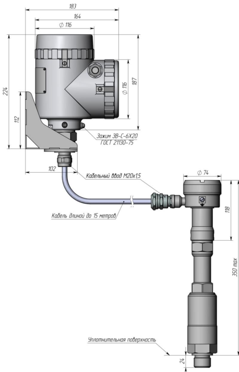
Рисунок Д93 - Габаритные и установочные размеры преобразователей с раздельным исполнением. Длина кабеля между блоком электронным и чувствительным элементом до 15 метров. Изоляторы ТЕГ. Работа при температуре до 500 °С. Способ присоединения – штуцер. Элемент чувствительный не показан
