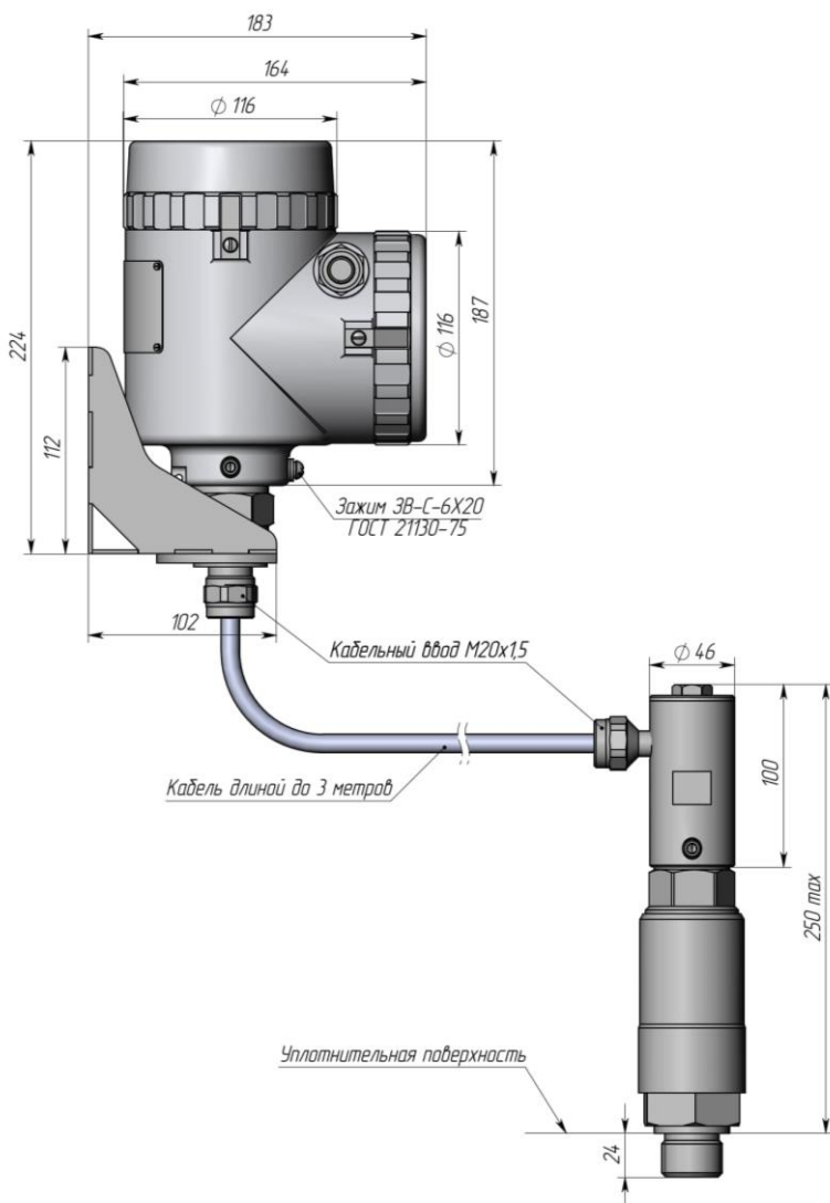
Рисунок Д83 - Габаритные и установочные размеры преобразователей с раздельным исполнением. Длина кабеля между блоком электронным и чувствительным элементом до 3 метров. Изоляторы TEG. Работа при температуре до 160 °С. Способ присоединения – штуцер. Элемент чувствительный не показан
