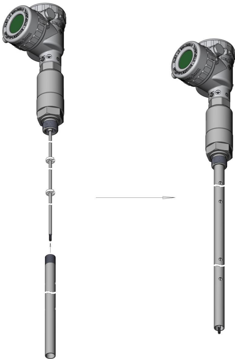
Рисунок М1.5 – Монтаж трубы из состава коаксиального зонда
