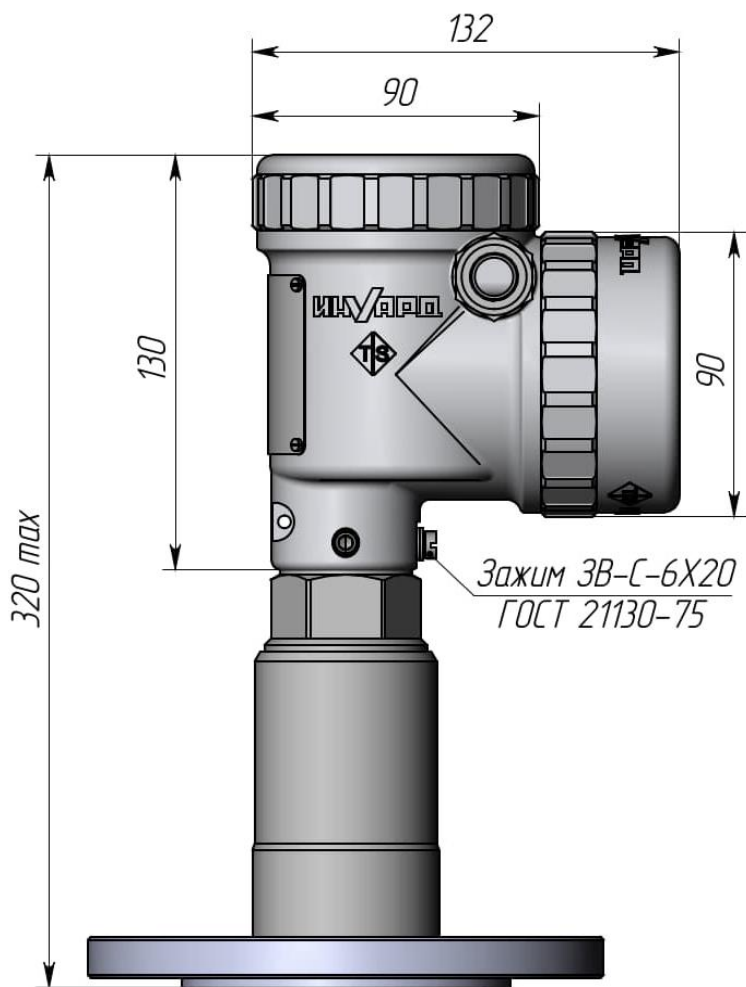
Рисунок Д103 - Габаритные и установочные размеры преобразователей с корпусом мини. Изоляторы ТЕГ. Работа при температуре до 160 °С. Способ присоединения – фланец. Элемент чувствительный не показан
