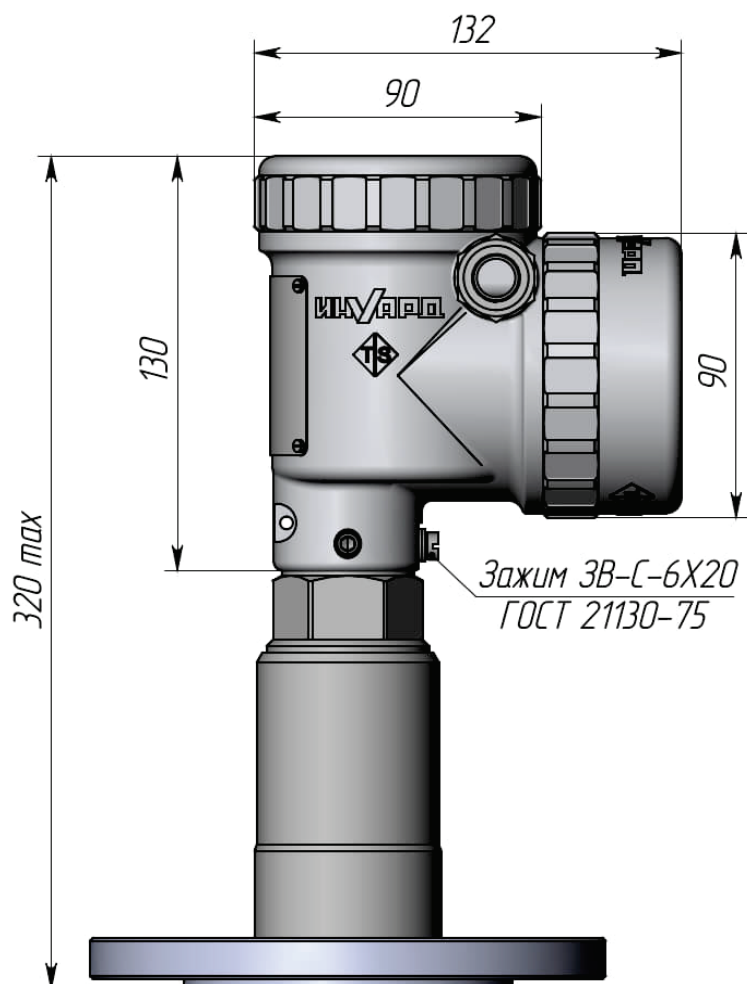
Рисунок Д103 - Габаритные и установочные размеры преобразователей с корпусом мини. Изоляторы ТEG. Работа при температуре до 160 °С. Способ присоединения – фланец. Элемент чувствительный не показан
