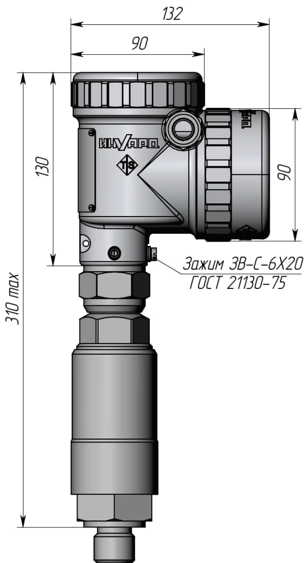
Рисунок Д100 - Габаритные и установочные размеры преобразователей с корпусом мини. Изоляторы ТЕР. Работа при температуре до 250 °С. Способ присоединения – штуцер. Элемент чувствительный не показан
