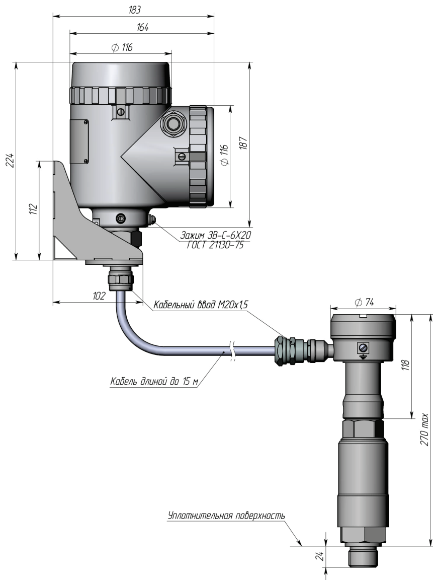
Рисунок Д91 - Габаритные и установочные размеры преобразователей с разделным исполнением. Длина кабеля между блоком электронным и чувствительным элементом до 15 метров. Изоляторы ТЕГ. Работа при температуре до 160 °С. Способ присоединения – штуцер. Элемент чувствительный не показан
