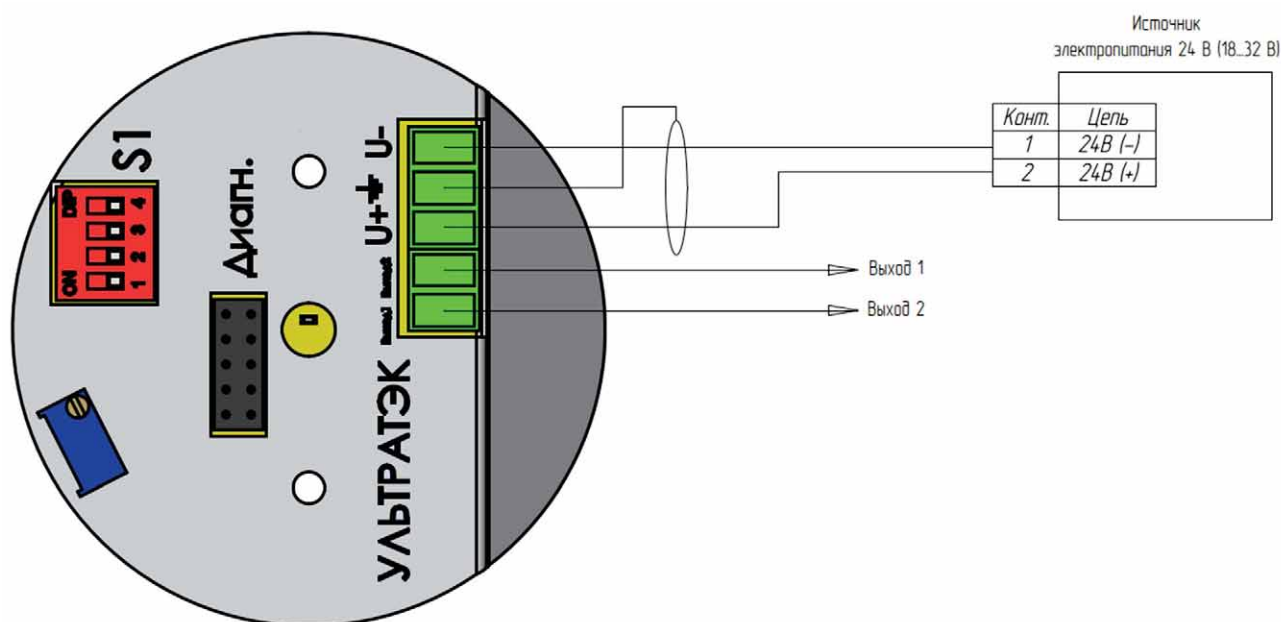
Рисунок 33 – Подключение кабеля к сигнализатору с двумя точками контроля, с релейным выходом 4-х проводная схема
