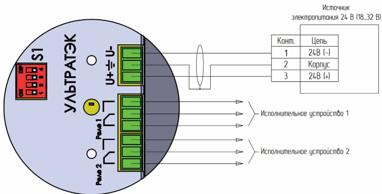
Рисунок 26 – Подключение сигнализатора исполнения P2 (РД)
