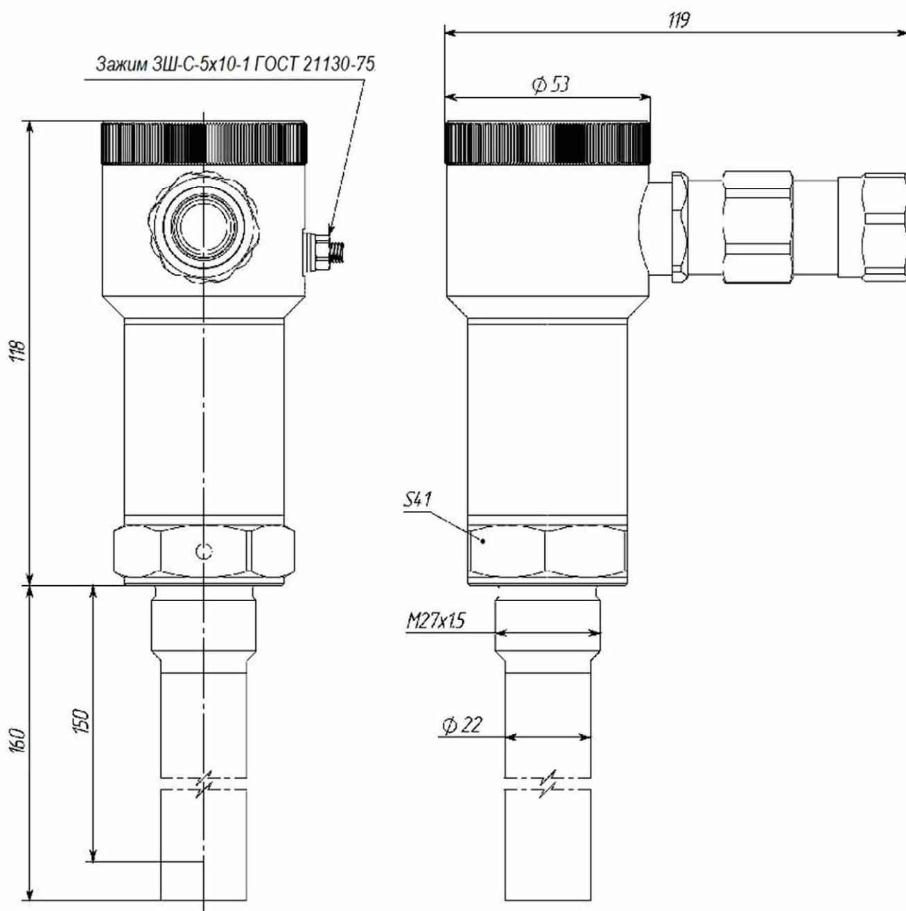
Рисунок Д.20 - Акустический датчик УЛЬТРАТЭК-С-М-Ж с одной точкой контроля для сред, находящихся при температуре не более 160 °С, присоединение к процессу – штуцер M27x1,5, G3/4, R3/4 с корпусом блока электронного третьего типа.
