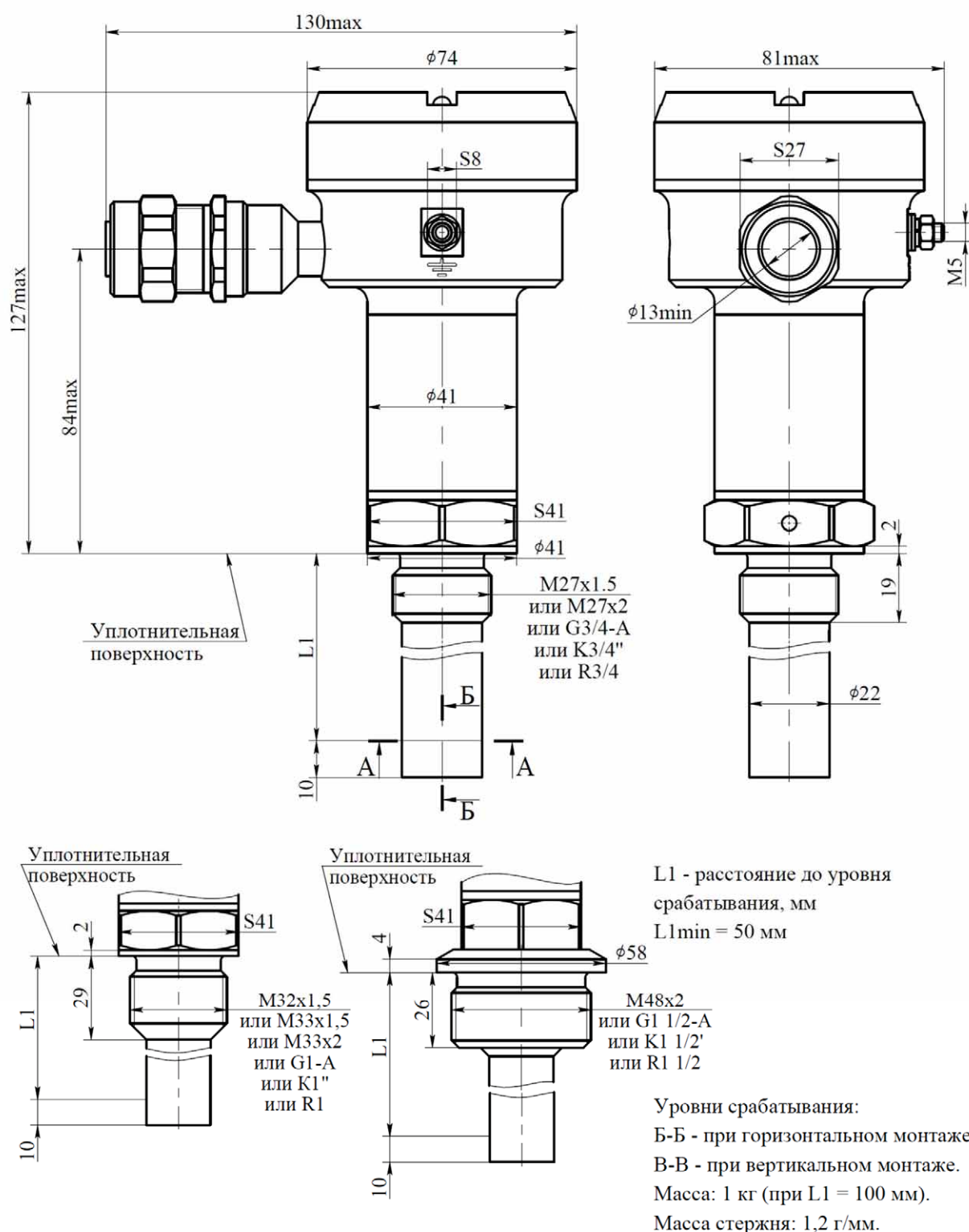
Рисунок Д.12 - Габаритные и установочные размеры акустического датчика УЛЬТРАТЭК-С-М-Ж с одной точкой контроля для сред, находящихся при температуре не более 160 °С, присоединение к процессу – штуцер.
