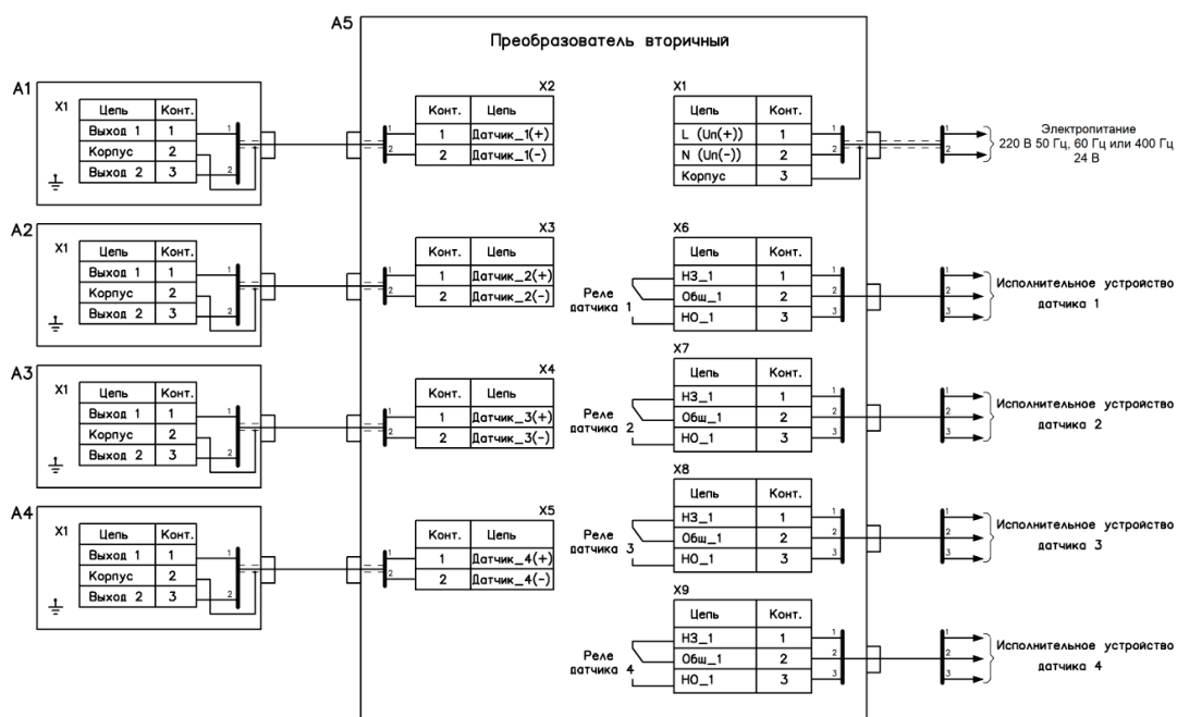
Рисунок Ж.6 - Схема электрическая подключения сигнализаторов с вторичным преобразователем ВП-22Х.
