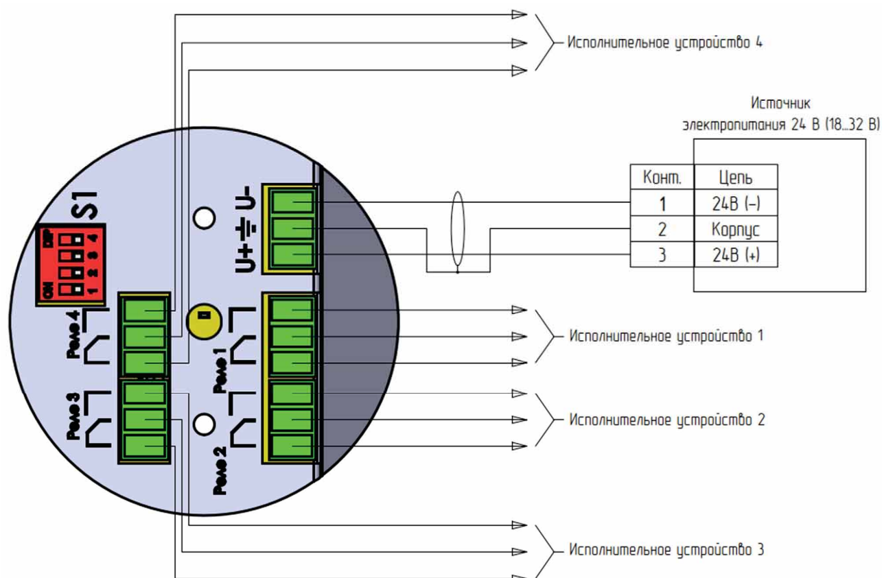
Рисунок 28 – Подключение сигнализатора исполнения Р4
