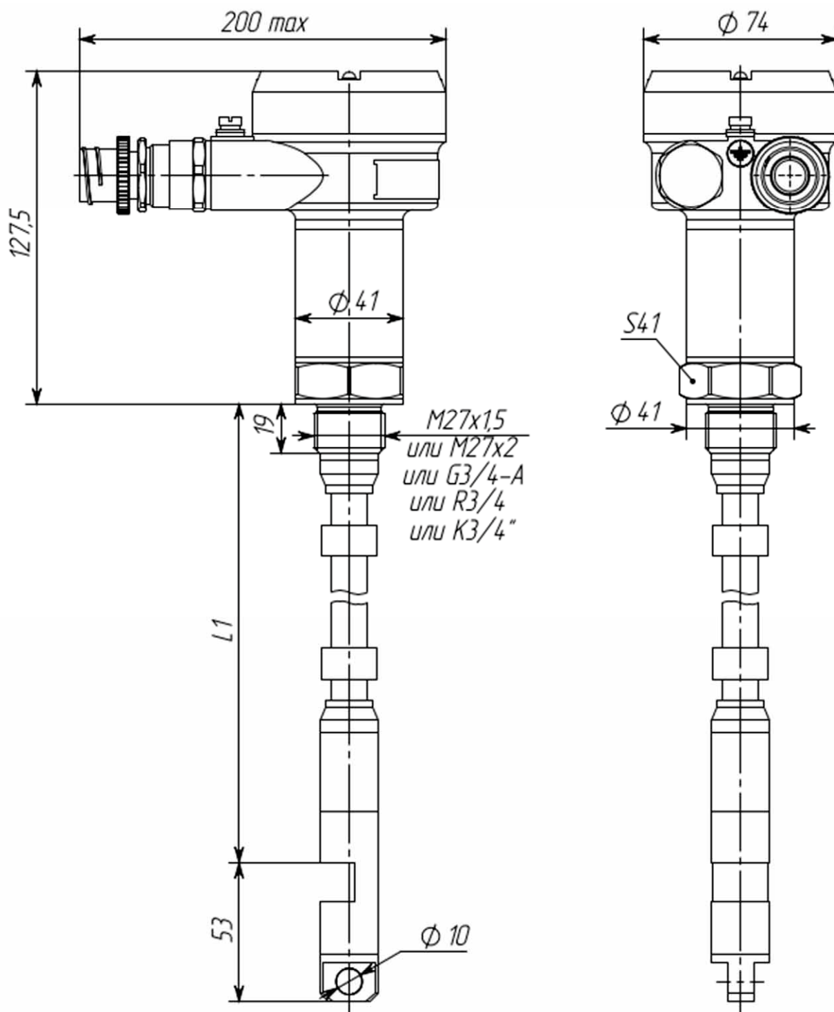
Рисунок Д.19 - Габаритные и установочные размеры акустического датчика УЛЬТРАТЭК-П-М-Г с одной точкой контроля для сред, находящихся при температуре не более 160 °С, присоединение к процессу – штуцер.
