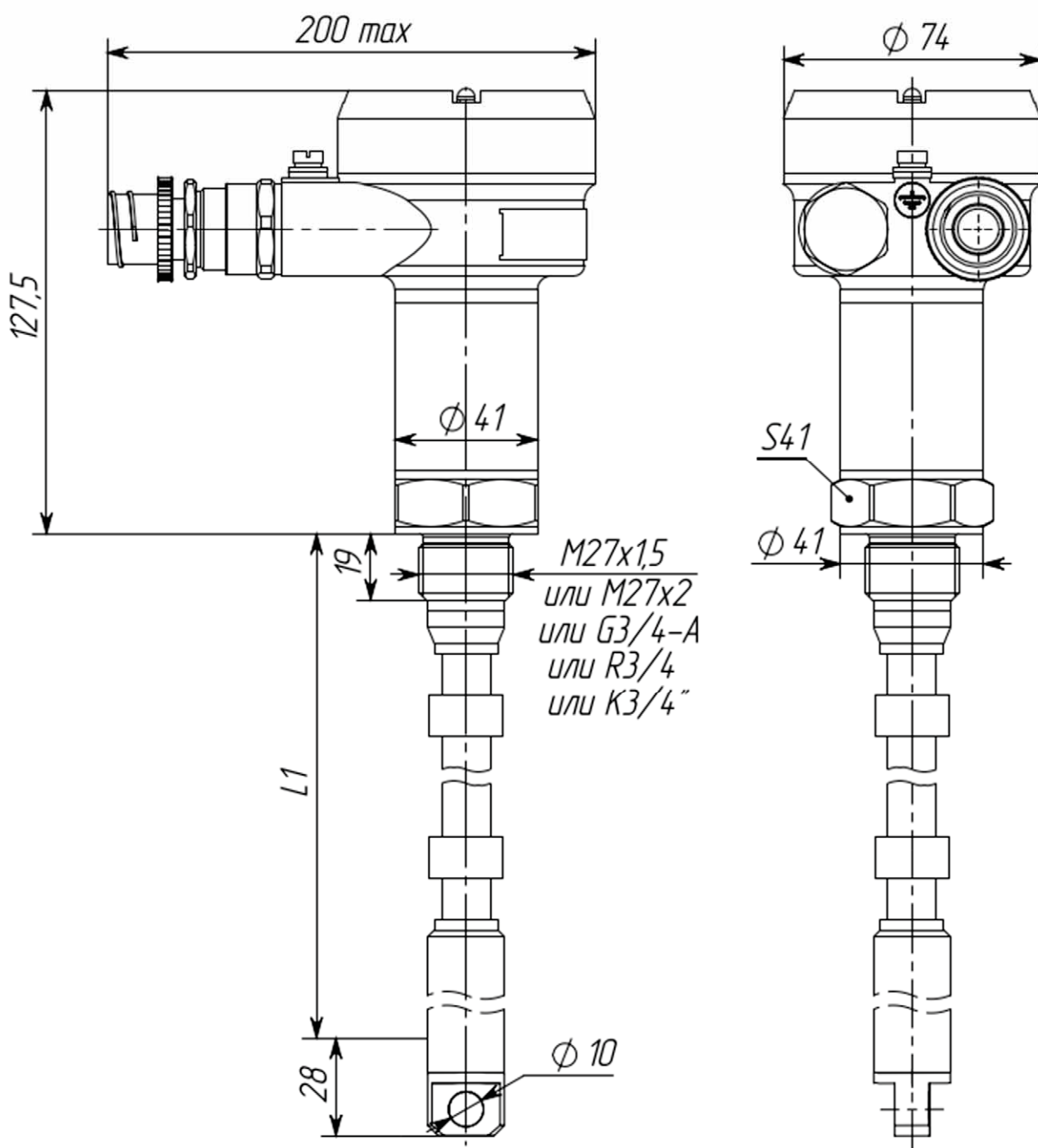
Рисунок Д.18 - Габаритные и установочные размеры акустического датчика УЛЬТРАТЭК-С-М-Г с одной точкой контроля для сред, находящихся при температуре не более 160 °С, присоединение к процессу – штуцер.
