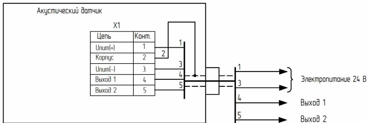
Рисунок Ж.11 – Схема подключения акустического датчика УЛЬТРАТЭК с двумя точками контроля, с релейным выходом 4-х проводная схема.
