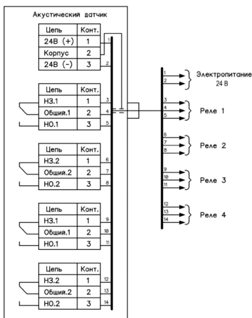
Рисунок Ж.3 - Схема электрическая подключения датчика с четырьмя выходными реле.
