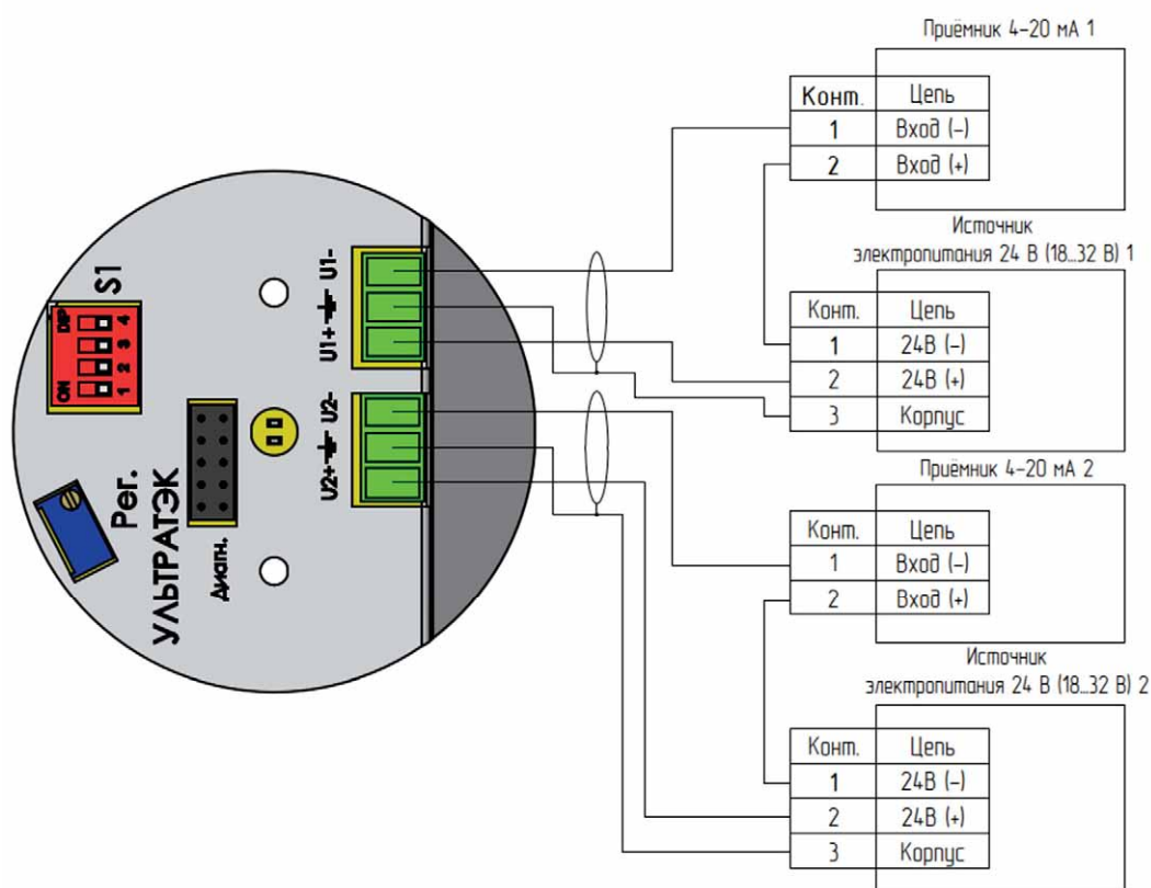
Рисунок 24 – Подключение сигнализатора исполнения 2А
