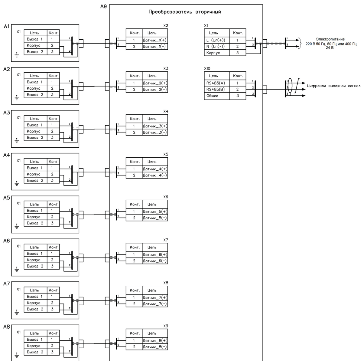
Рисунок Ж.9 - Схема электрическая подключения сигнализаторов УЗС-6Т с вторичным преобразователем ВП-88Х с цифровым выходным сигналом.
