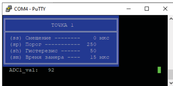
Рисунок К.2 - Отладочная информация прибора в PuTTY
