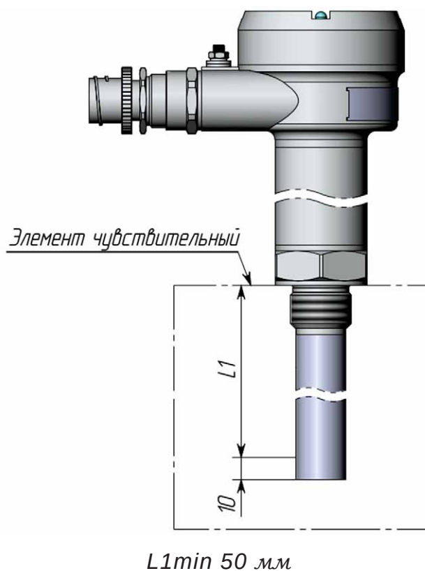
Рисунок 13 – Конструкция ультразвукового сигнализатора уровня со стержневым сенсором УЛЬТРАТЭК-С
