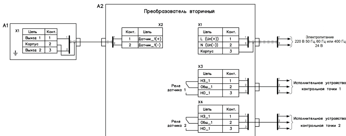
Рисунок Ж.5 - Схема электрическая подключения сигнализаторов с вторичным преобразователем ВП-12Х.
