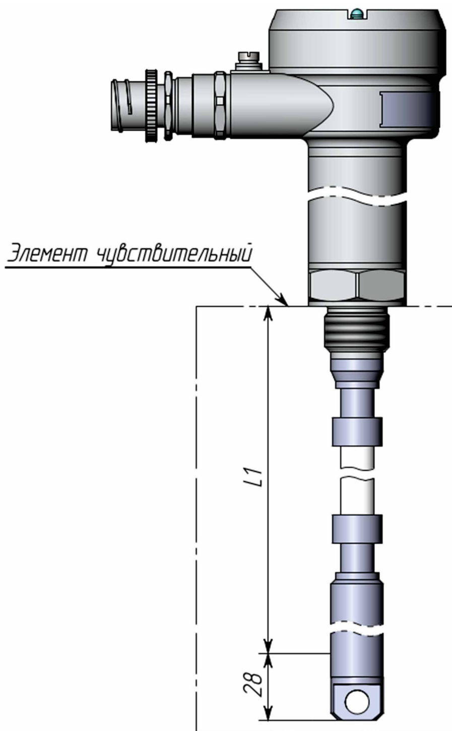
Рисунок 15 – Конструкция ультразвукового сигнализатора уровня с гибким стержневым сенсором
