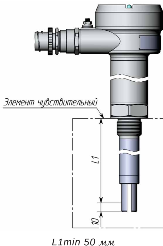
Рисунок 14 – Конструкция ультразвукового сигнализатора уровня с вилочным сенсором УЛЬТРАТЭК-В
