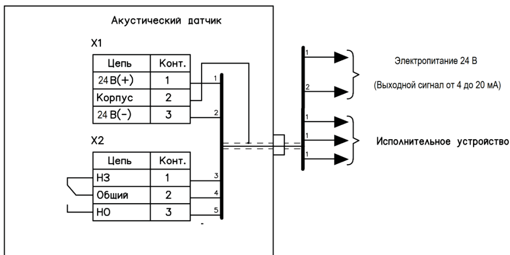
Рисунок Ж.1 - Схема электрическая подключения датчиков (к системе верхнего уровня или вторичному преобразователю).
