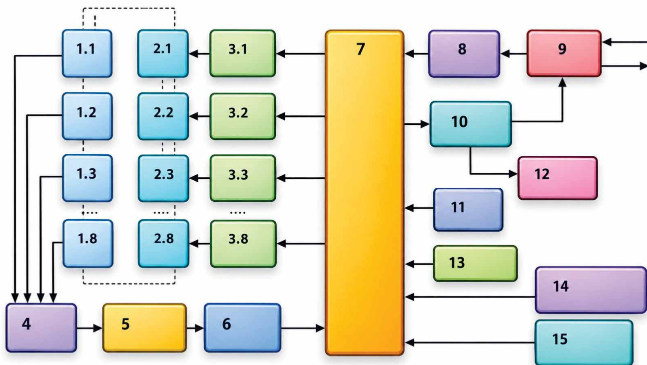
Рисунок 2 - Структурная схема акустического датчика
