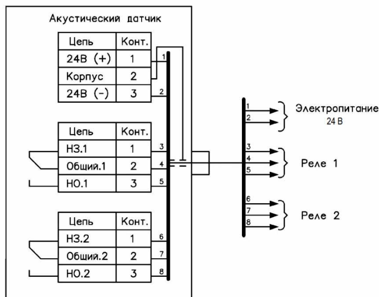
Рисунок Ж.2 - Схема электрическая подключения датчика с двумя выходными реле.
