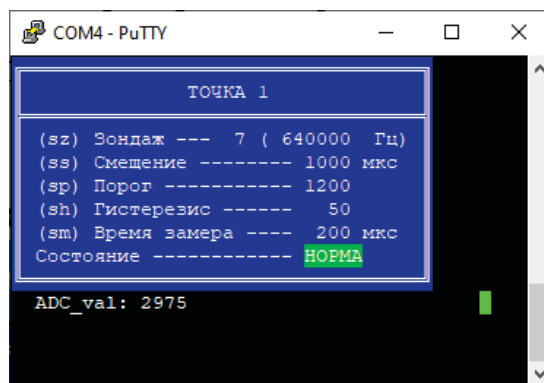
Рисунок И.2 - Отладочная информация прибора в PuTTY
