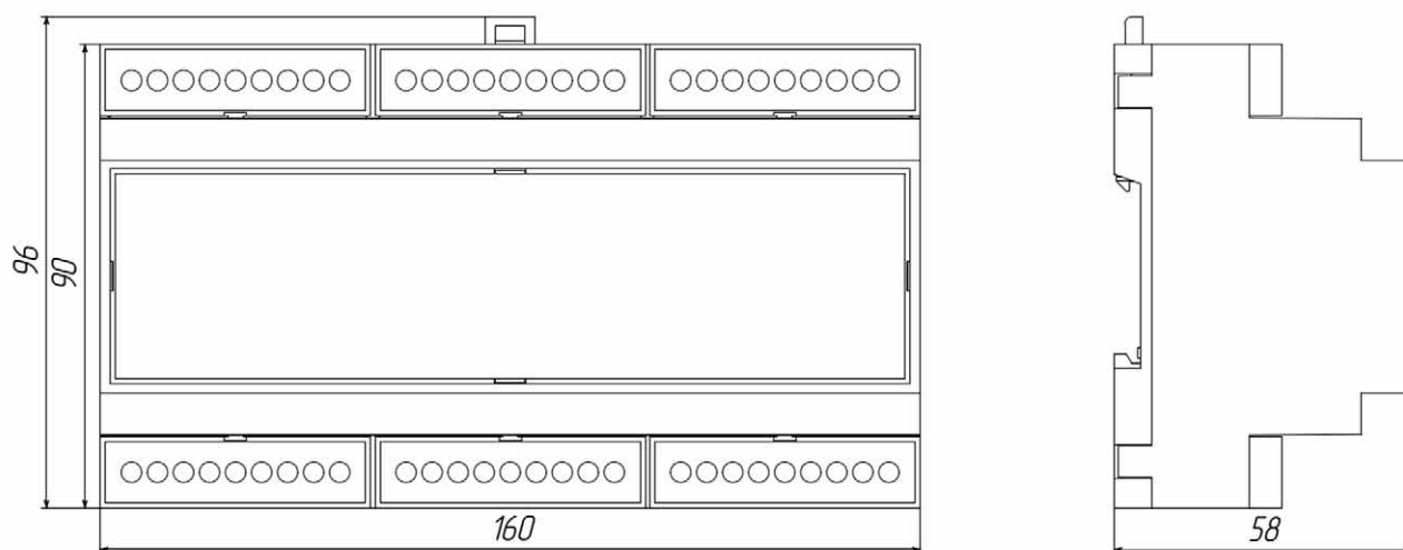
Рисунок Е.3 - Габаритные и установочные размеры вторичного преобразователя для четырех датчиков со степенью защиты корпуса IP20 по ГОСТ 14254 - 2015 и креплением на DIN-рейку.
