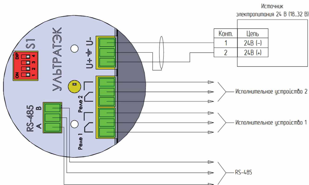
Рисунок 30 – Подключение кабеля к сигнализатору исполнения ЦС+P2
