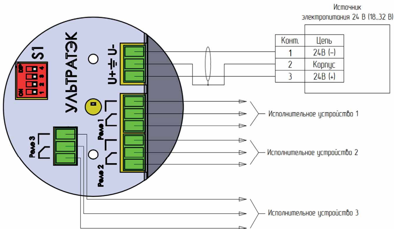
Рисунок 27 – Подключение сигнализатора исполнения P3
