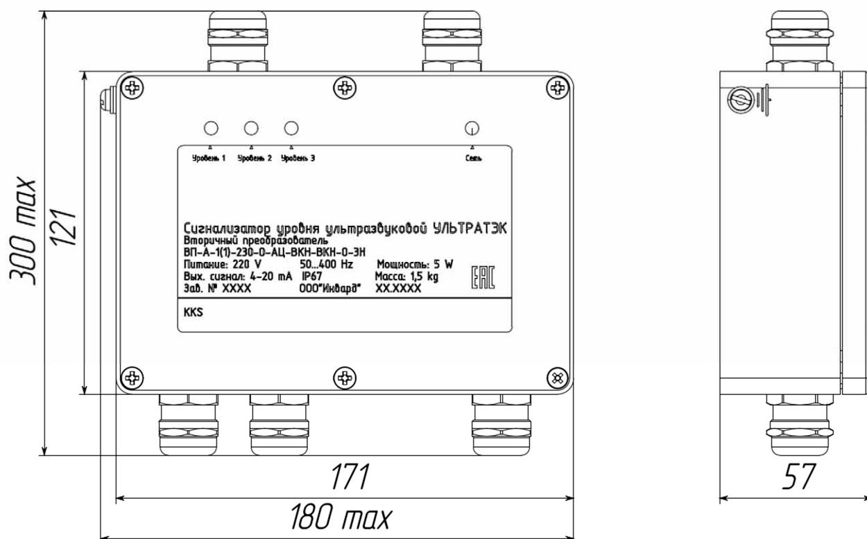
Рисунок Е.4 - Габаритные и установочные размеры вторичного преобразователя для четырех датчиков со степенью защиты корпуса IP67 по ГОСТ 14254 - 2015
