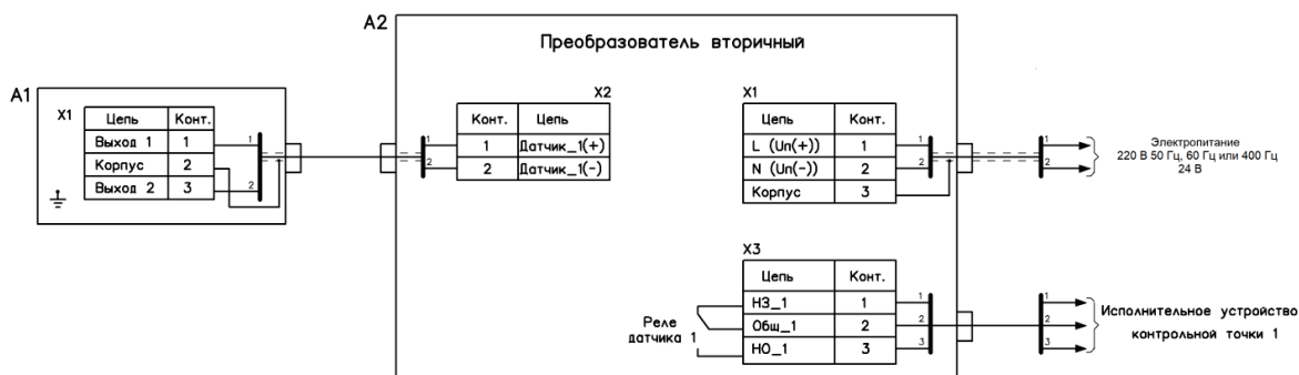
Рисунок Ж.4 - Схема электрическая подключения сигнализаторов с вторичным преобразователем ВП-11Х.
