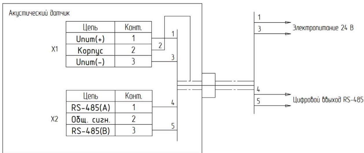
Рисунок Ж.10 – Схема подключения акустического датчика УЛЬТРАТЭК с выходом RS-485 с протоколом MODBUS RTU
