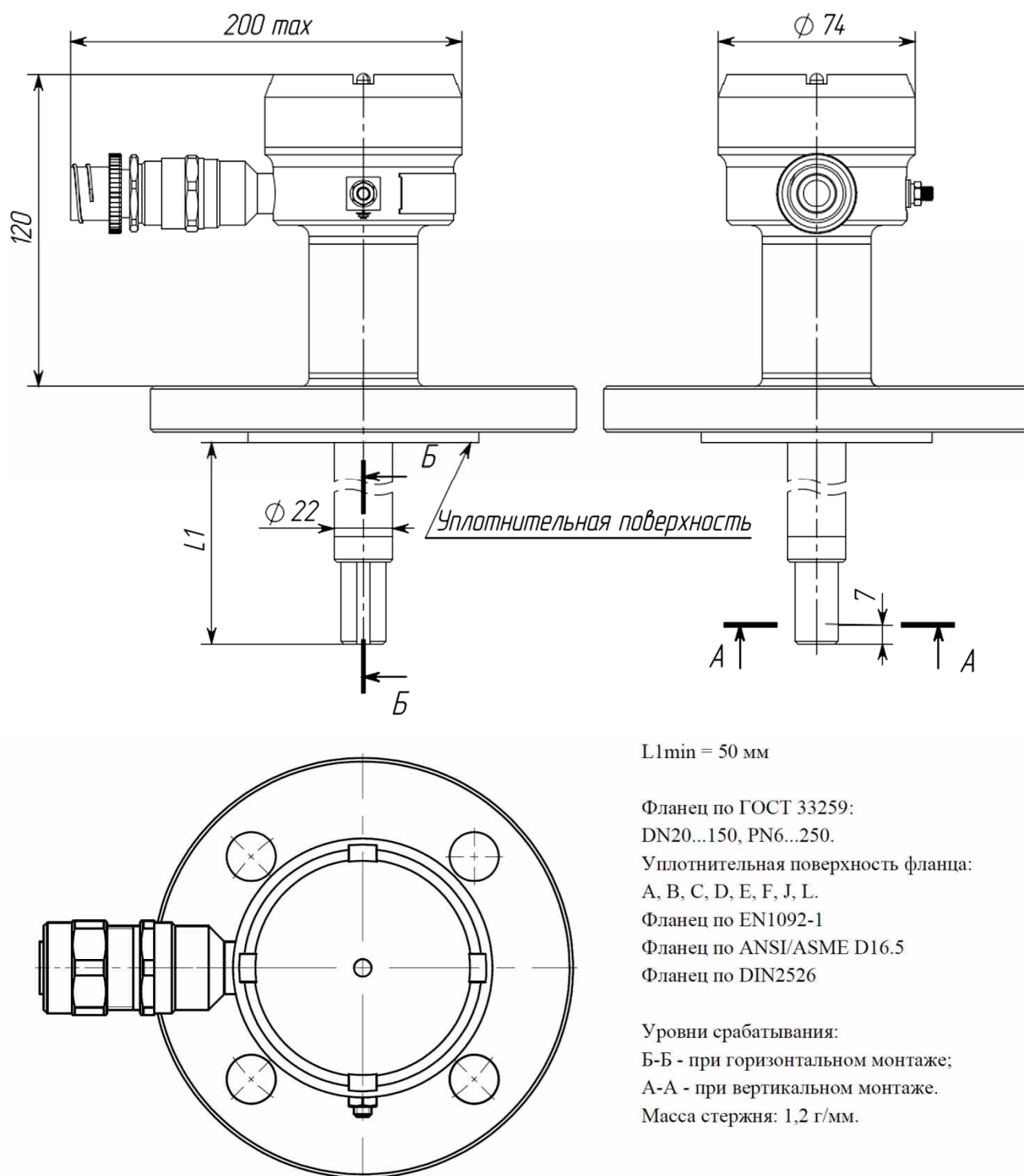
Рисунок Д.11 - Габаритные и установочные размеры акустического датчика УЛЬТРАТЭК-В-М-Ж с одной точкой контроля для сред, находящихся при температуре не более 160 °С, присоединение к процессу – фланец.
