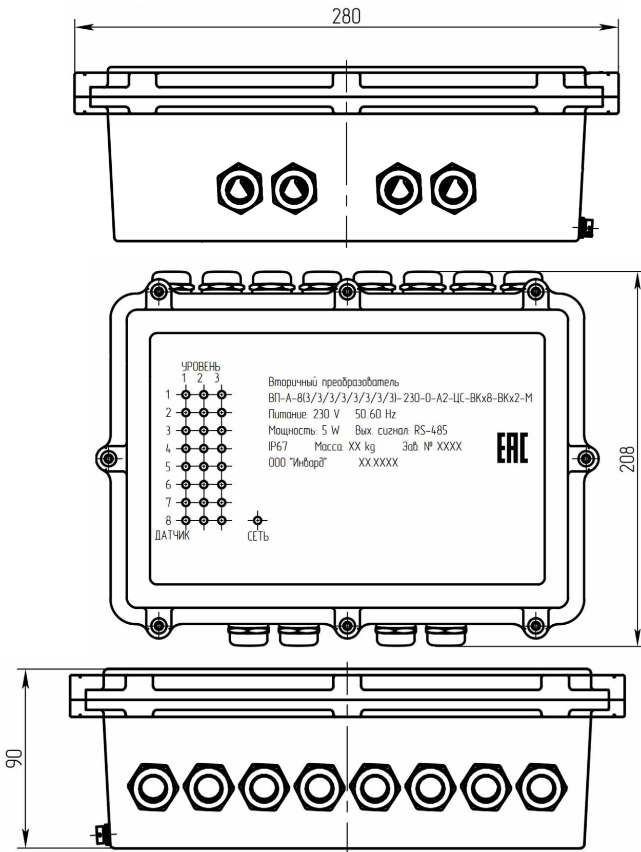
Рисунок Е.5 - Габаритные и установочные размеры вторичного преобразователя для восьми датчиков со степенью защиты корпуса IP67 по ГОСТ 14254 - 2015
