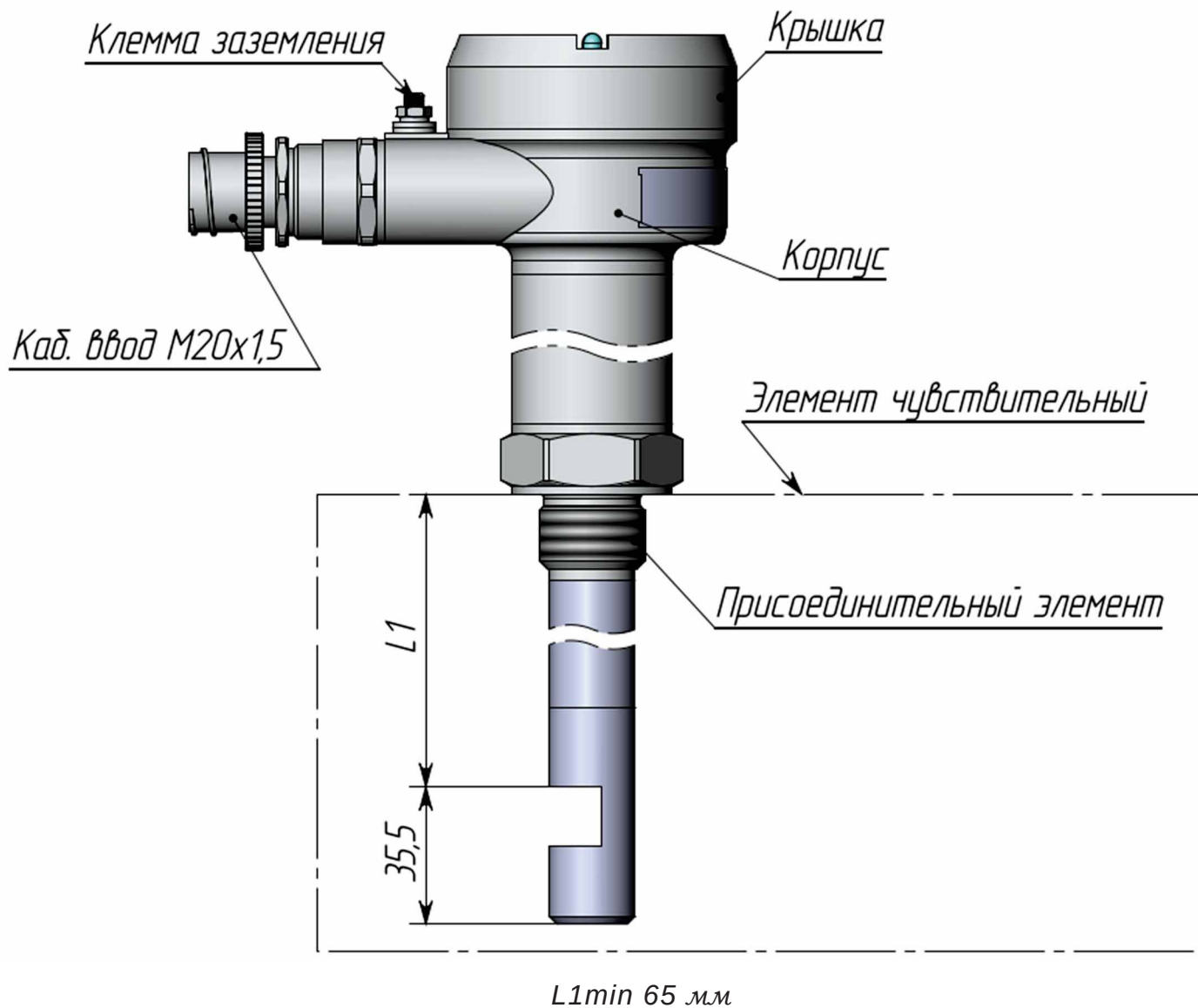
Рисунок 12 – Конструкция ультразвукового сигнализатора уровня с просветным сенсором УЛЬТРАТЭК-II
