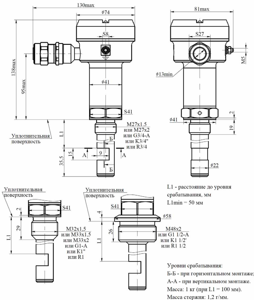
Рисунок Д.1 - Габаритные и установочные размеры акустического датчика УЛЬТРАТЭК-П-М-Ж с одной точкой контроля для сред, находящихся при температуре не более 160 °С, присоединение к процессу – штуцер, корпус блока электронного первого типа с одним кабельным вводом.
