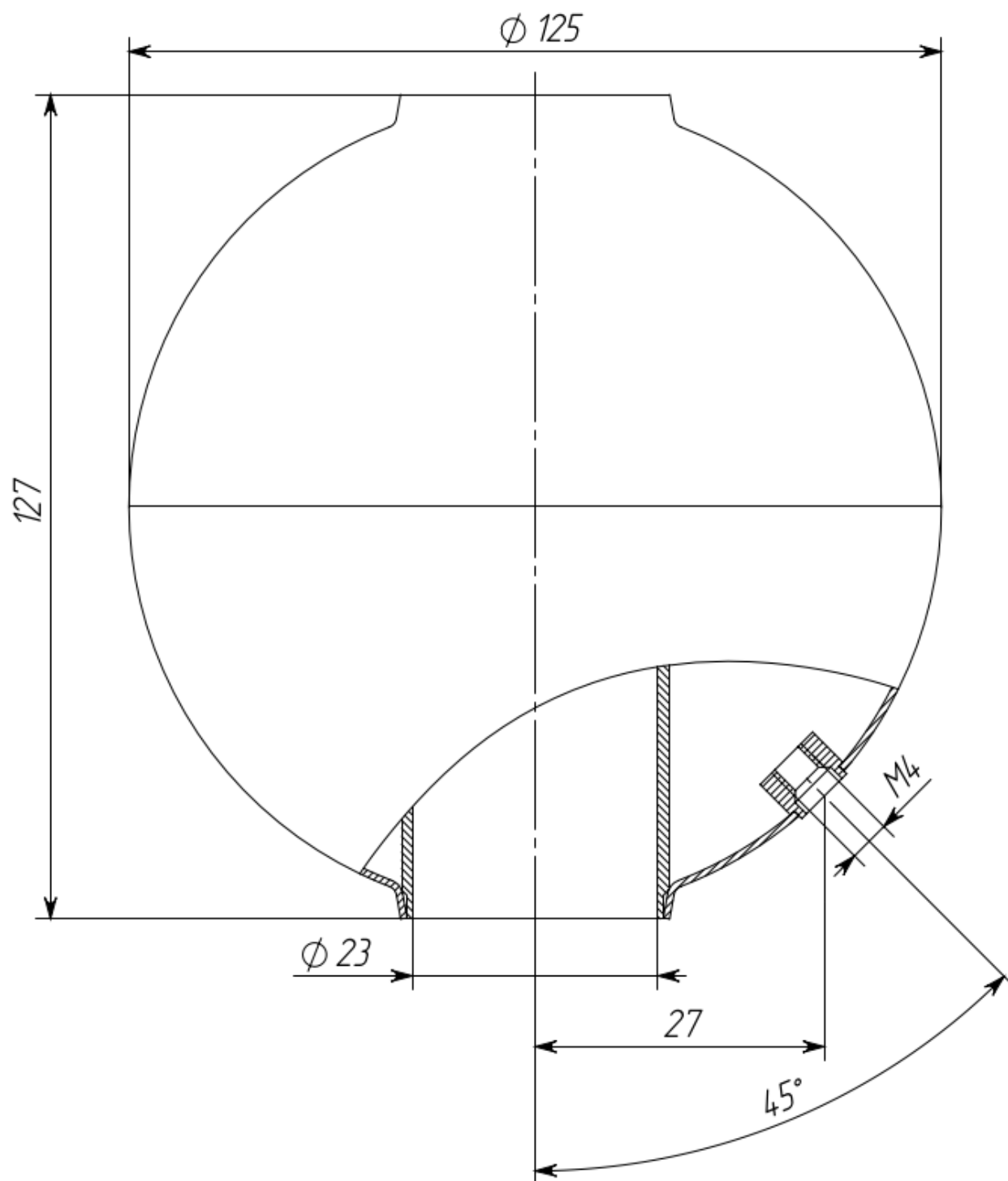
Рисунок Е.2 – Габаритные и установочные размеры поплавка Н125 (масса 220 г)
