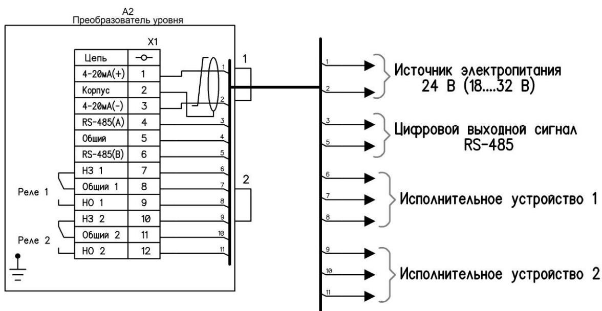
Рисунок Ж.5 – Схема электрическая подключения преобразователей исполнения 485
