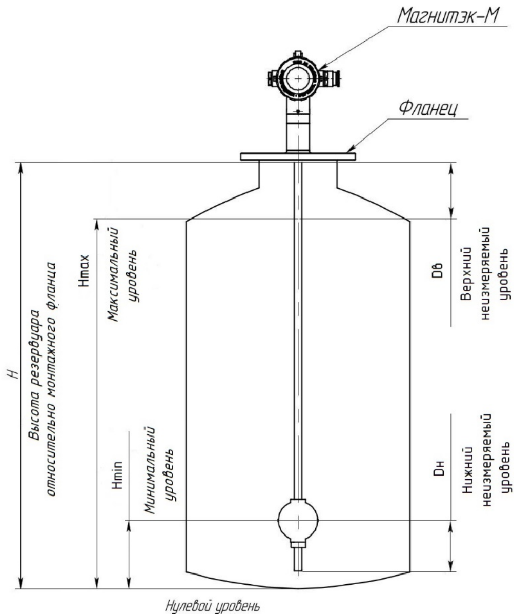
Рисунок К.5 – Пояснения к вводу параметров прибора с фланцевым или резьбовым соединением с резервуаром.
