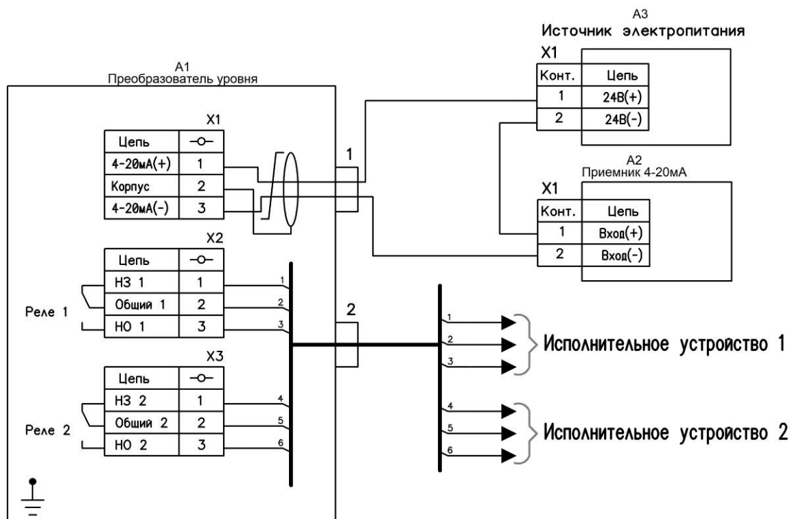
Рисунок Ж.4 – Схема электрическая подключения преобразователей исполнения АР без местного индикатора
