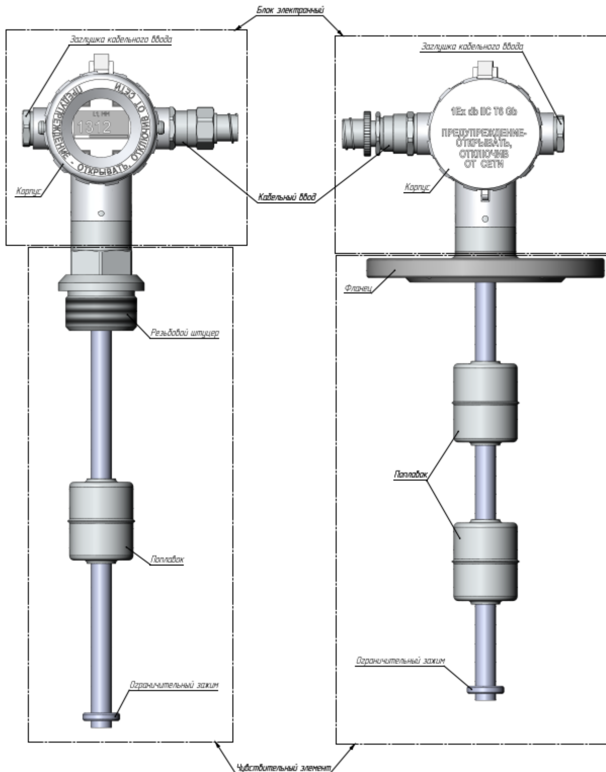
Рисунок 2 – Устройство преобразователя
