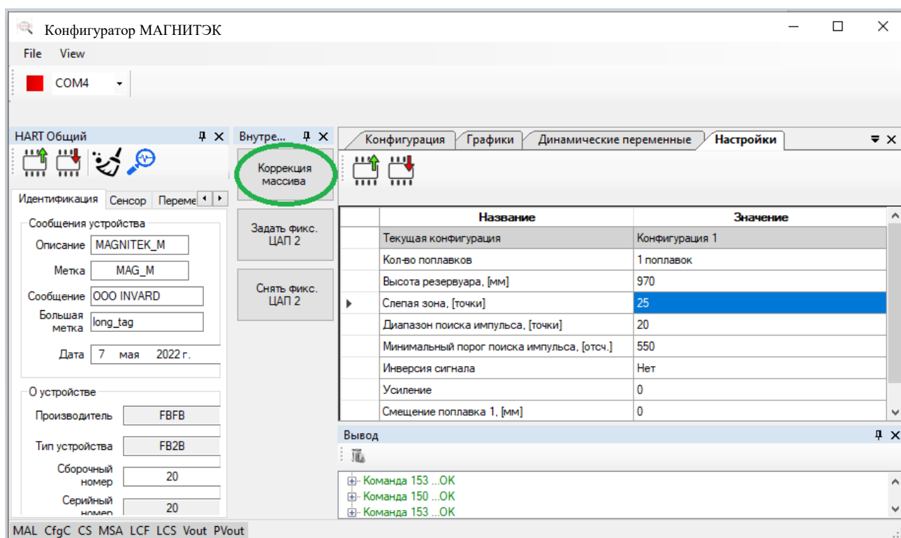
Рисунок 18 - Коррекция массива
