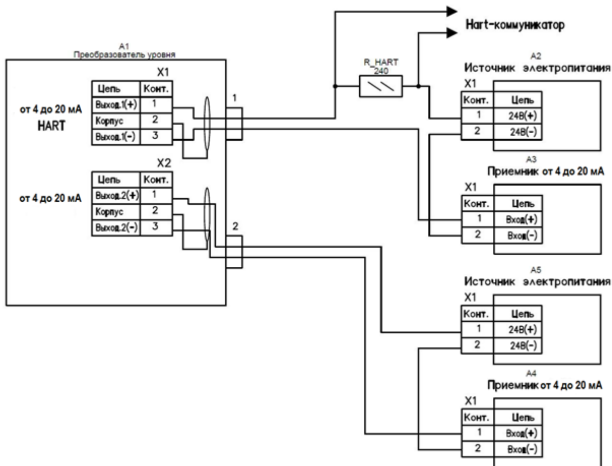
Рисунок Ж.8 – Схема электрическая подключения преобразователей исполнения А2Ц
