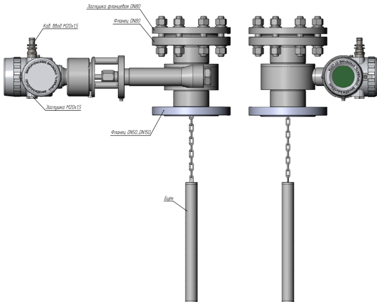
Рисунок 4 – Преобразователь со способом присоединения через фланец
