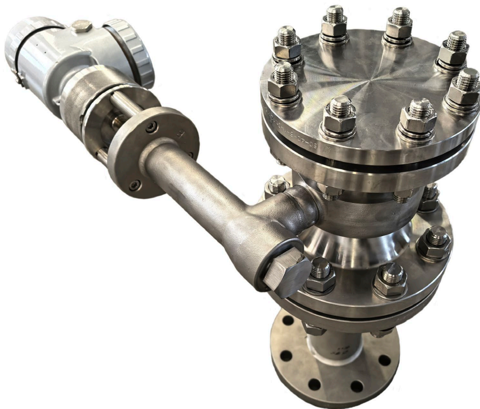
Рисунок 13 – Установка заглушки-фланца
