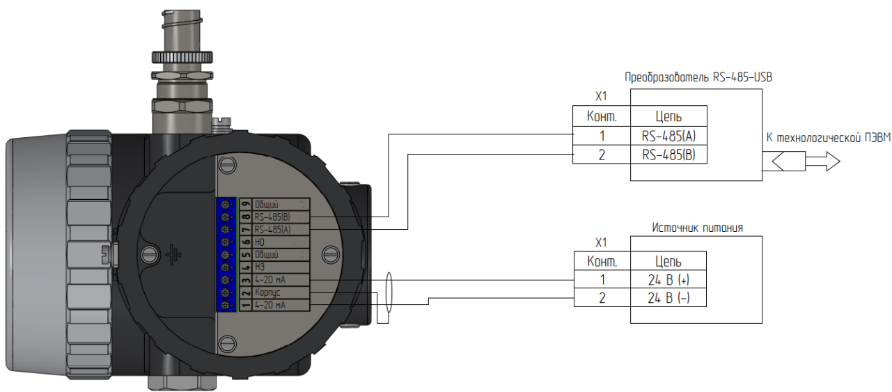
Рисунок 18 – Подключение кабеля к преобразователю исполнения ЦС
