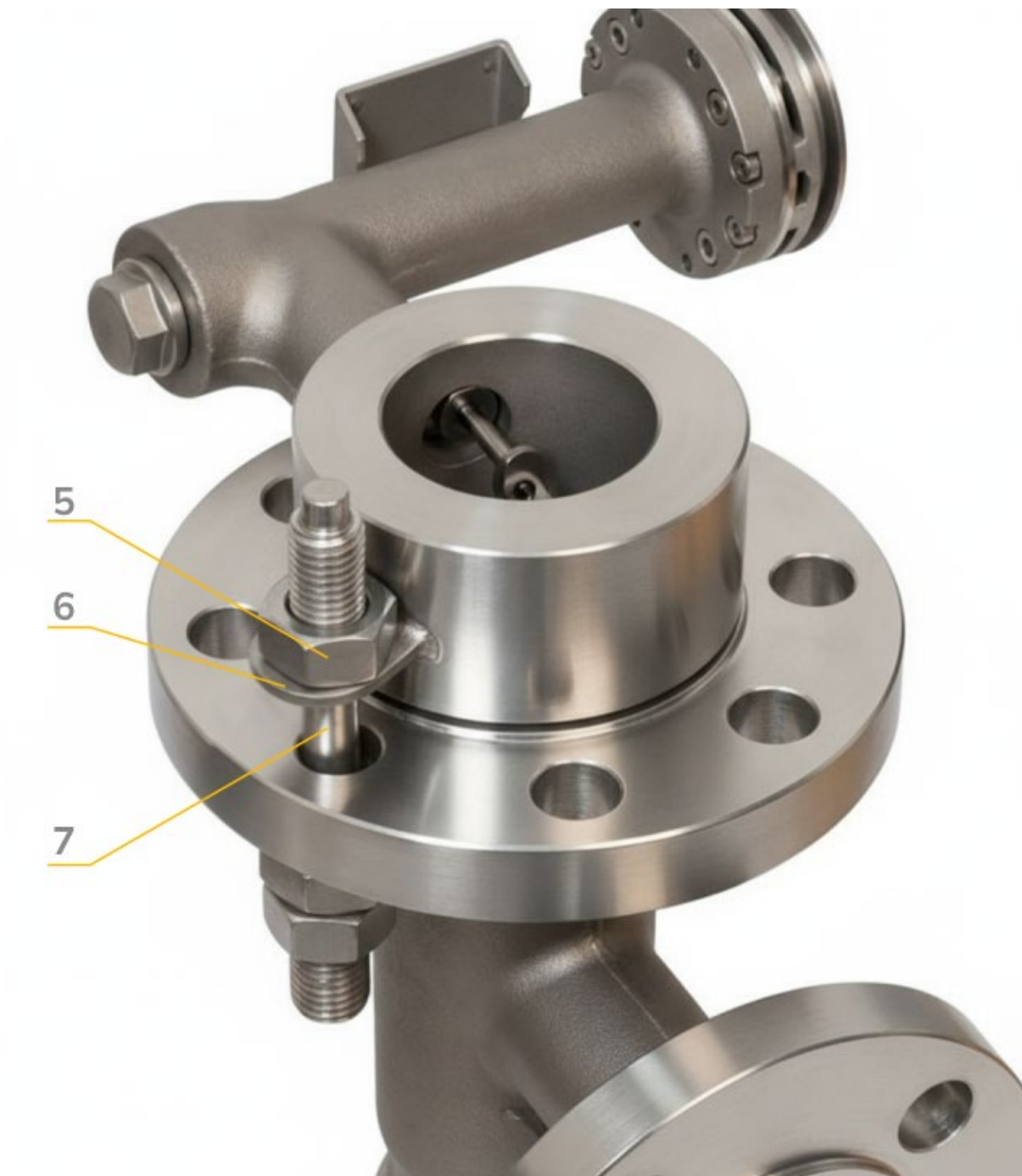
Рисунок 10 – Установка преобразователя на соединительный фланец
