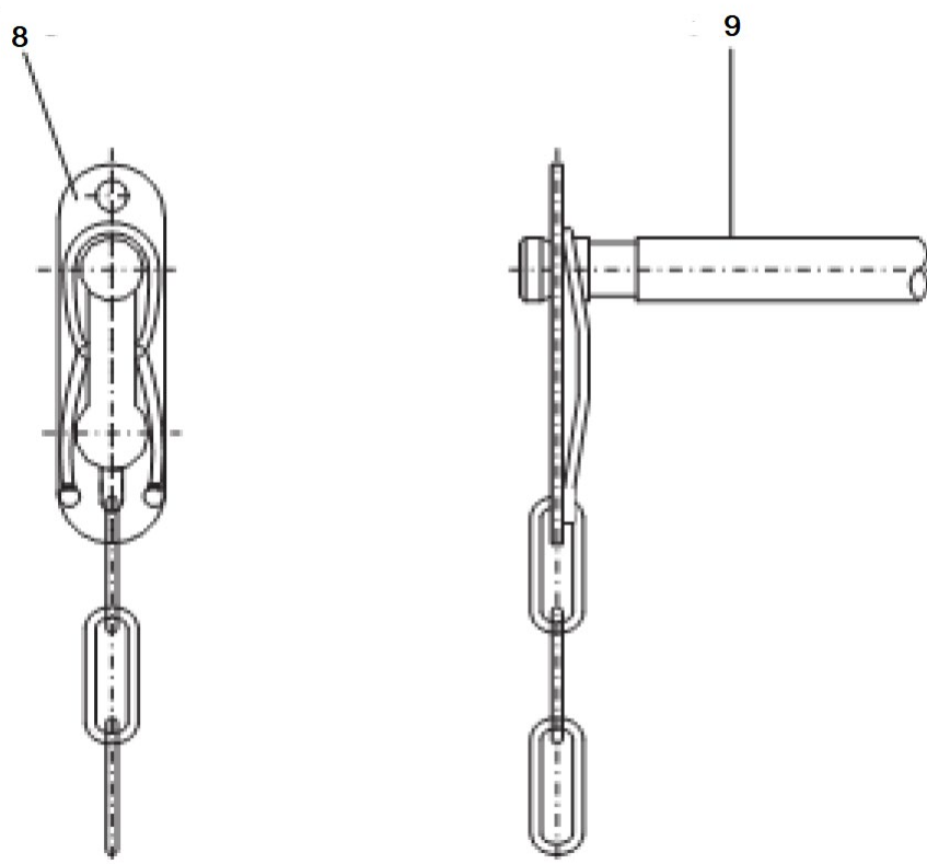
Рисунок 14 – Монтаж цепи
