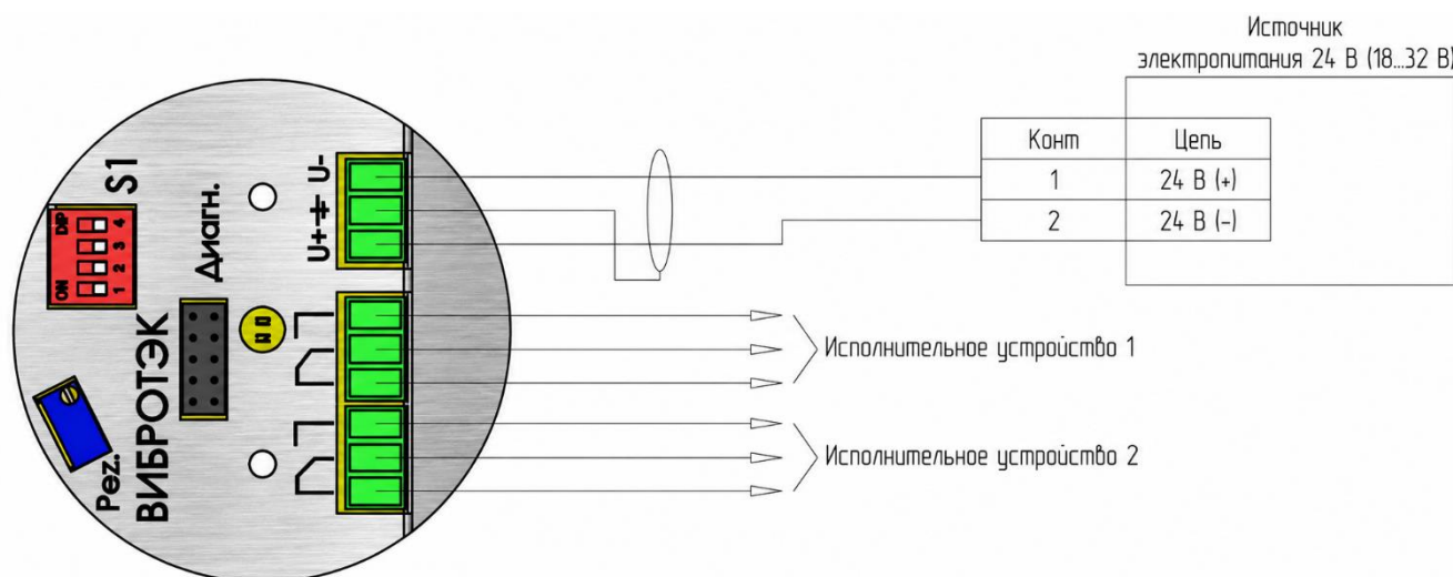
Рисунок 41 – Схема подключения специального исполнения В450 и для сыпучей среды (Р1)
