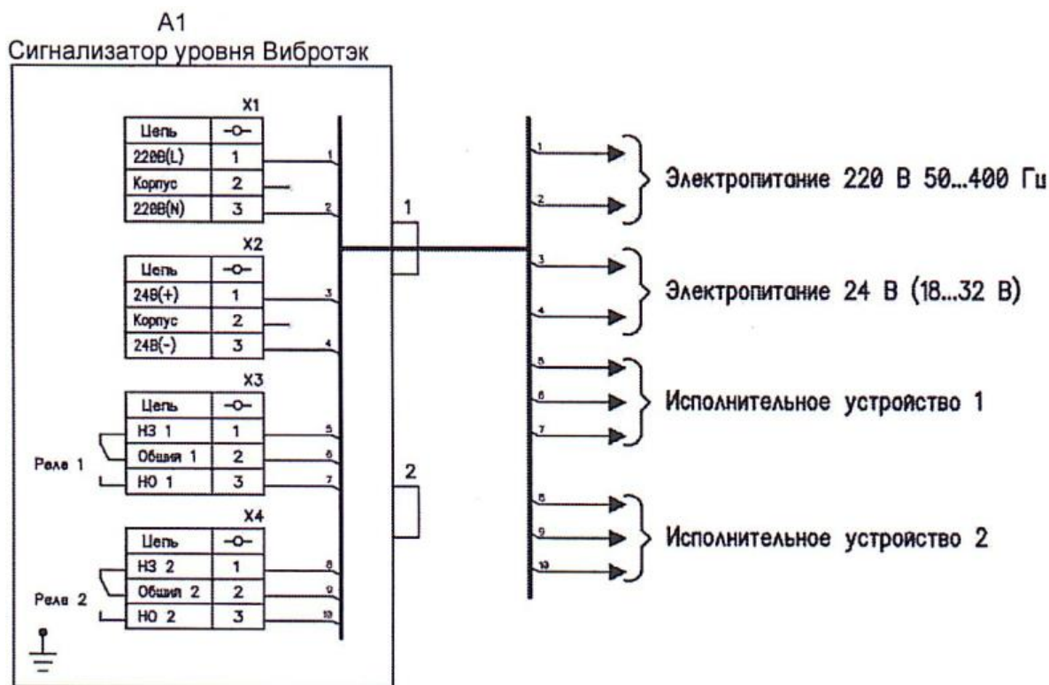
Рисунок Д.3 – Схема электрическая подключения сигнализатора с выходными релейными сигналами Р1, Р2, РР, РД
