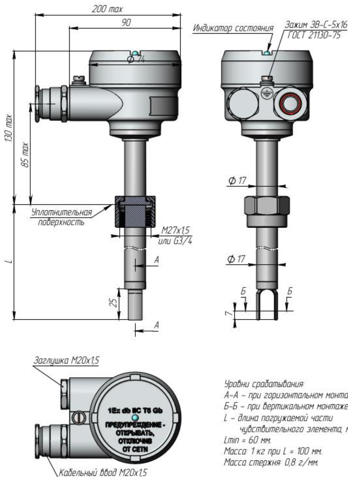
Рисунок В.37 – Габаритные и установочные размеры сигнализатора уровня ВИБРОТЭК-У-М-В со способом присоединения накидная гайка M27x1,5, G3/4 для работы при температурах контролируемой среды не более 100 °С
