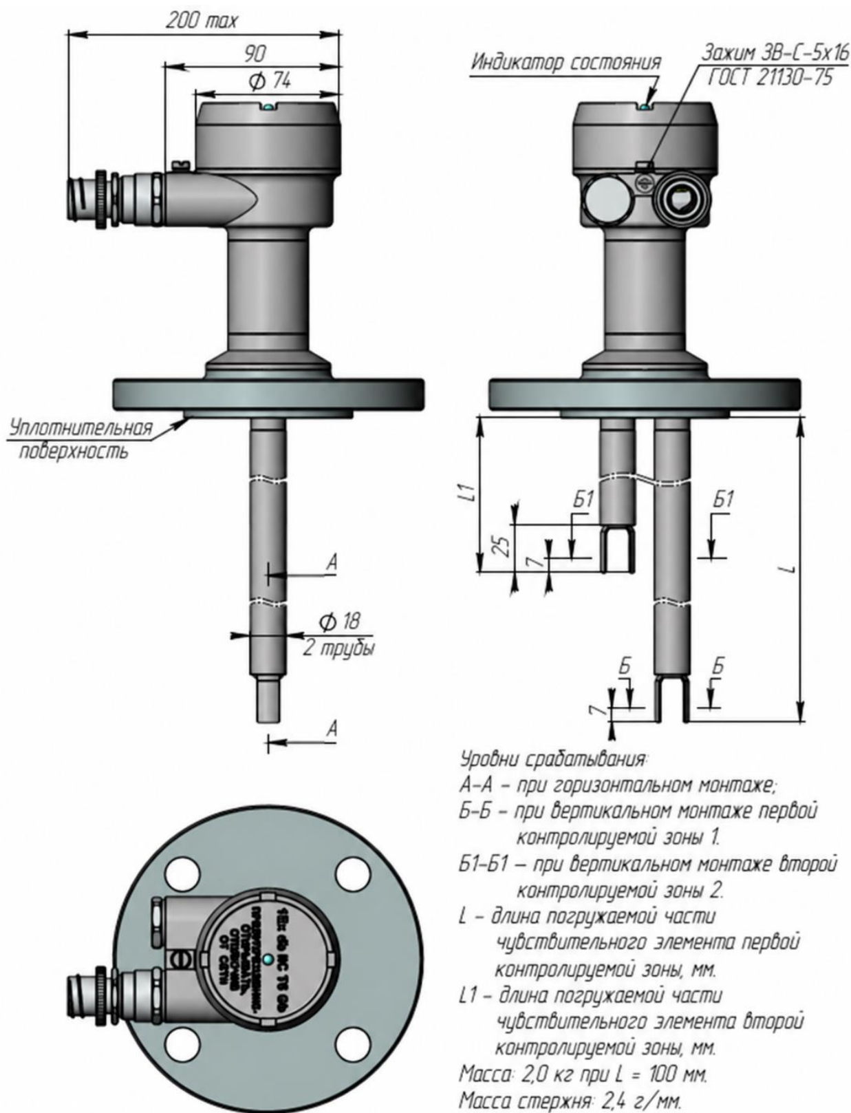
Рисунок В.42 – Габаритные и установочные размеры сигнализатора уровня ВИБРОТЭК-У-М-В с двумя точками контроля. Способ присоединения – фланец, температура контролируемой среды не более 160 °С
