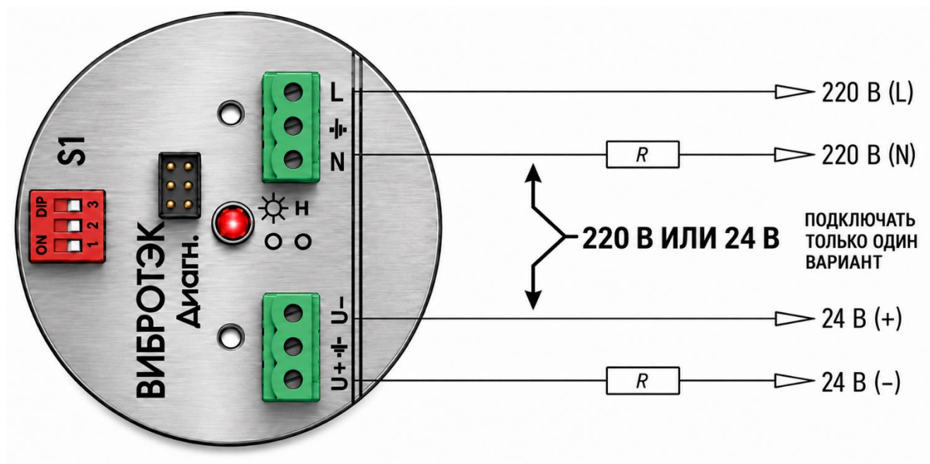
Рисунок 34 – Подключение сигнализатора исполнения БК (220 В и/или 24 В)
