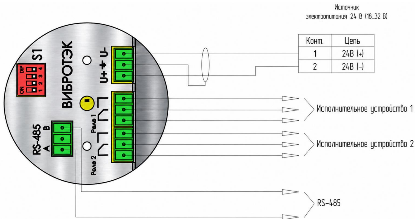
Рисунок 35 – Подключение сигнализатора исполнения ЦС с выходным сигналом по интерфейсу RS-485 и двумя выходными релейными сигналами
