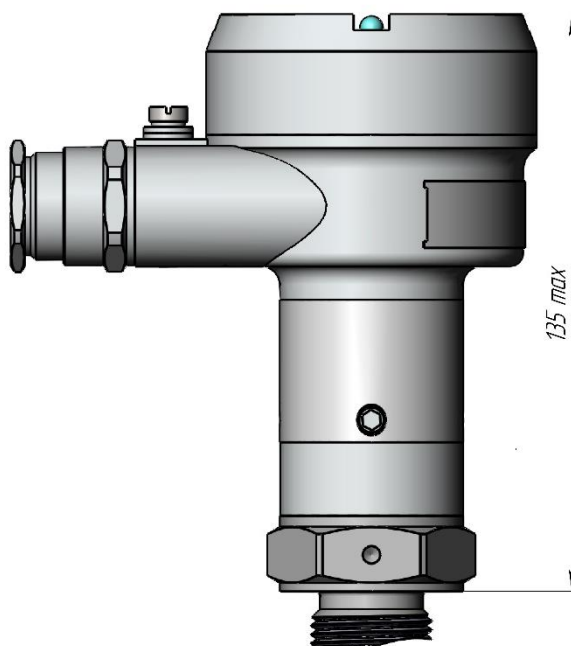
Рисунок В.14 – Габаритные размеры перехода на 160 °С (100 °С) с поворотным механизмом
