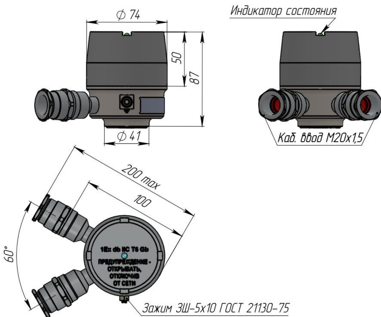
Рисунок В.6 – Габаритные размеры корпуса блока электронного в корпусе из нержавеющей стали для оборудования класса безопасности 3Н (высокая крышка, два кабельных ввода)
