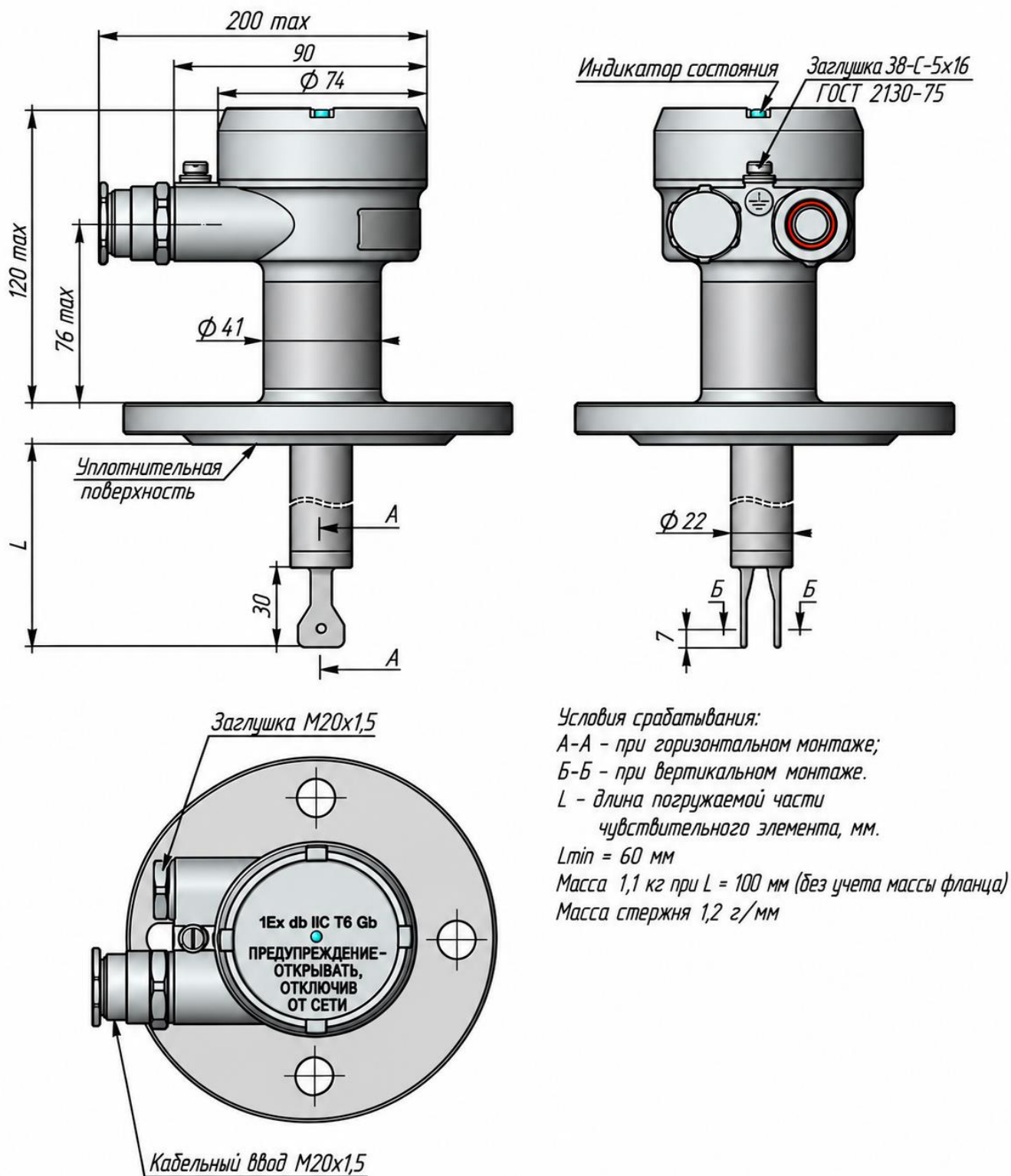
Рисунок В.35 – Габаритные и установочные размеры сигнализатора уровня ВИБРОТЭК-У-М-В исполнения В100, В160 и В250 со способом присоединения фланец для работы при температурах контролируемой среды не более 160 °С
