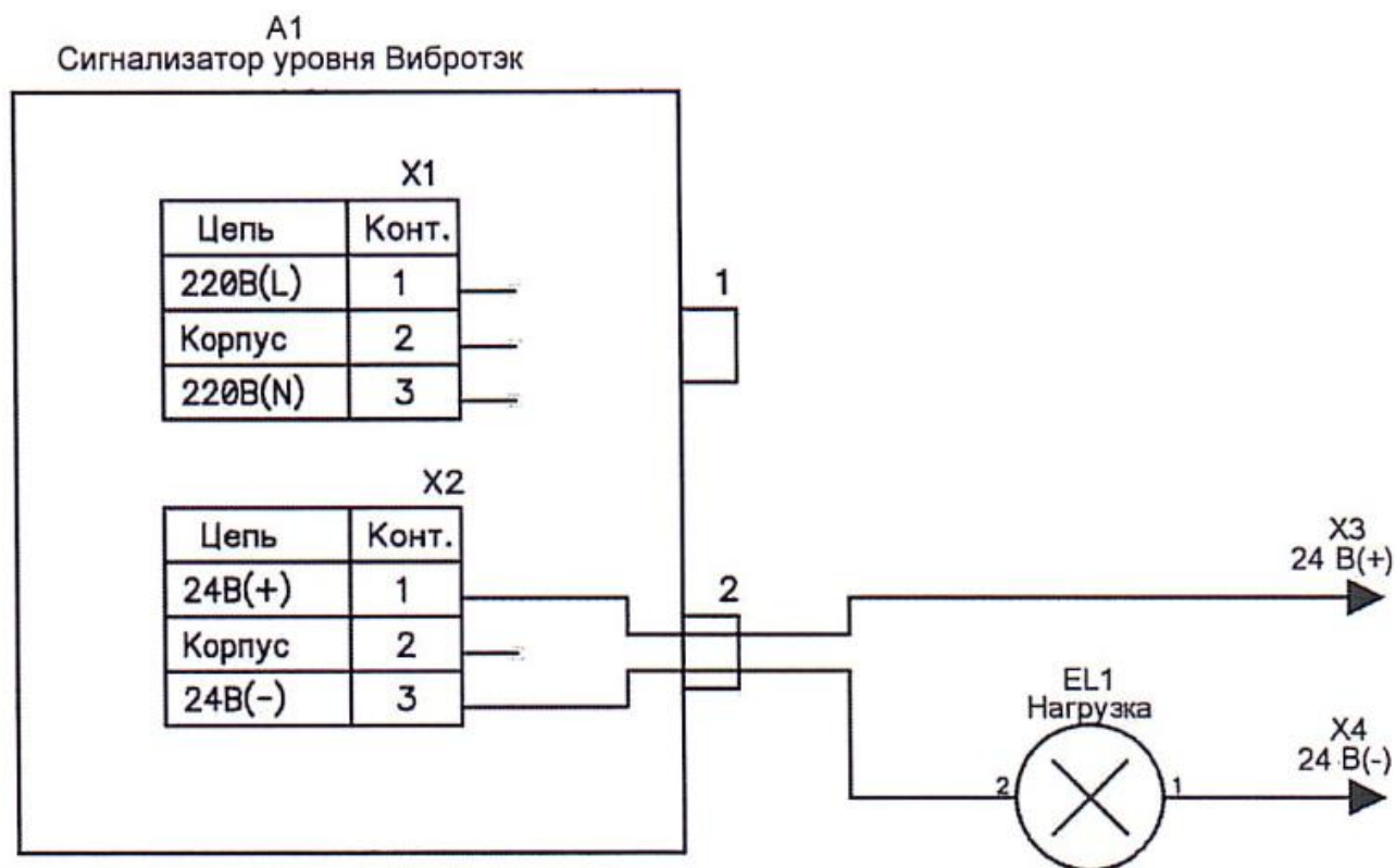
Рисунок Д.13 – Схема электрическая подключения сигнализатора с выходным сигналом БК с электропитанием напряжением постоянного тока 24 В
