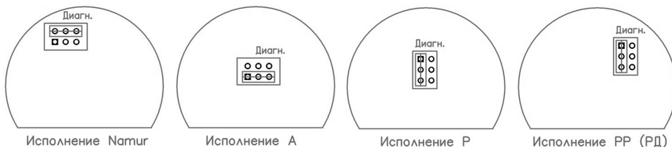
Рисунок 44 – Положение перемычки при переключении сигнализаторов в режим «Настройка порога»
