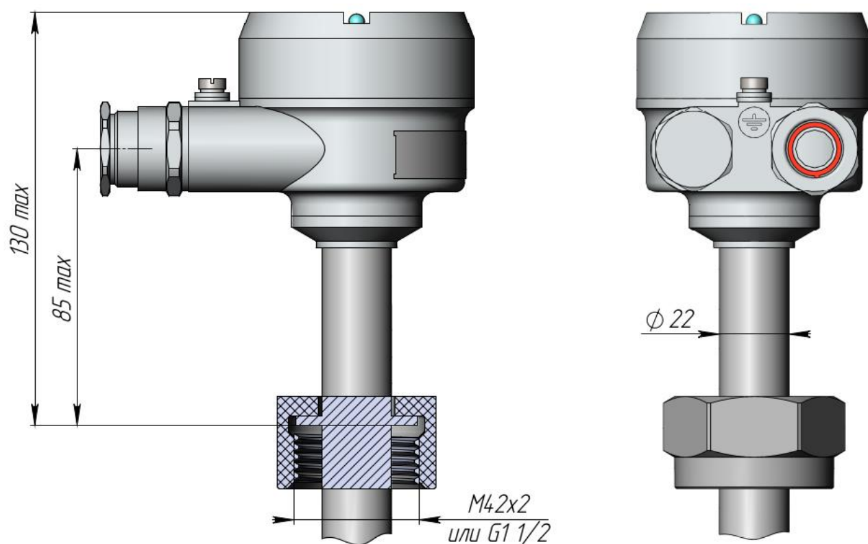
Рисунок В.17 – Габаритные размеры перехода на 100 °С с накидной гайкой
