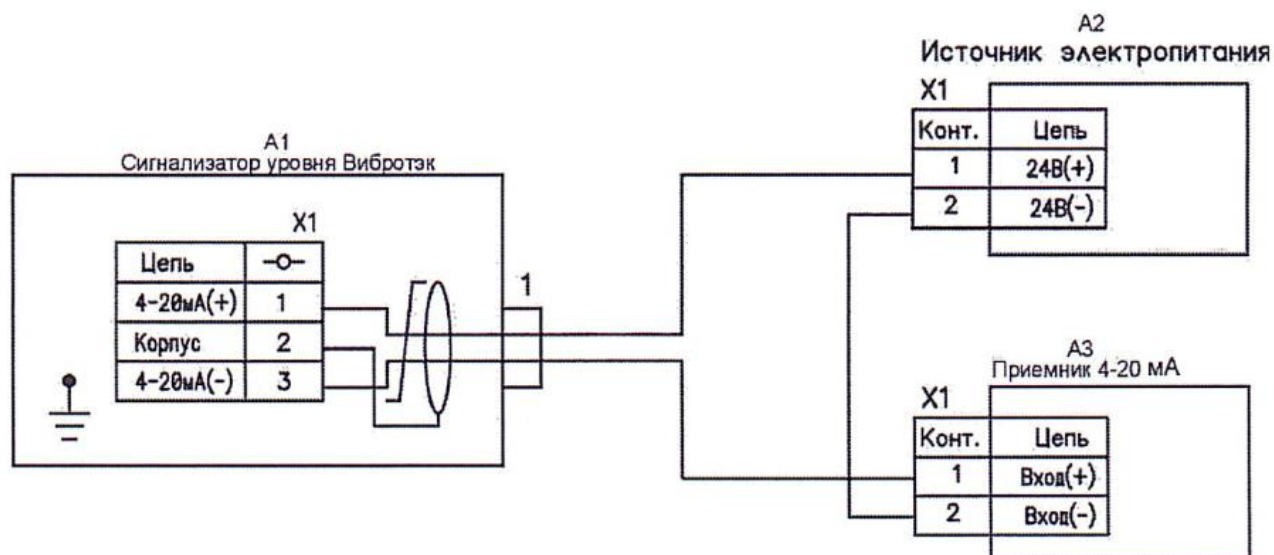
Рисунок Д.1 – Схема электрическая подключения сигнализатора с выходными сигналами A1, A2, A3
