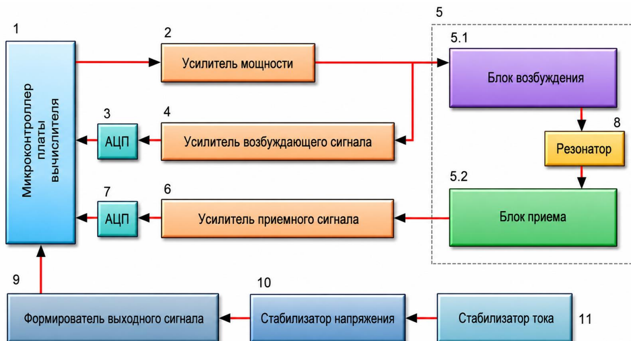
Рисунок 3 – Структурная схема сигнализаторов
