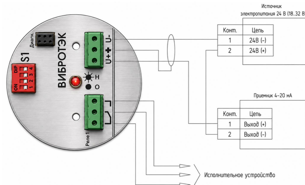
Рисунок 31 – Подключение сигнализатора исполнения Р2, РД, РР (220 В/24 В)
