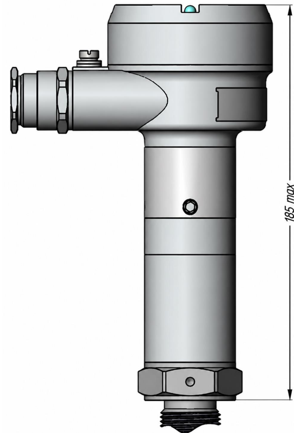
Рисунок В.15 – Габаритные размеры перехода на 250 °С с поворотным механизмом (или газонепроницаемый)
