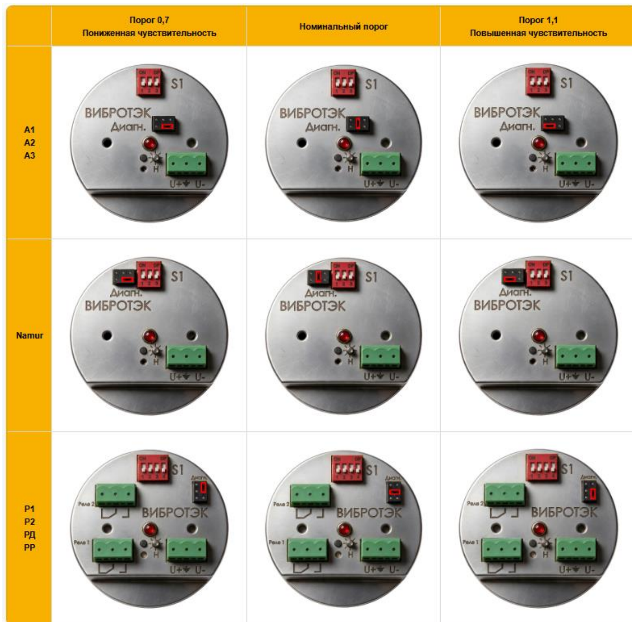
Рисунок 59 – Изменение чувствительности сигнализатора
