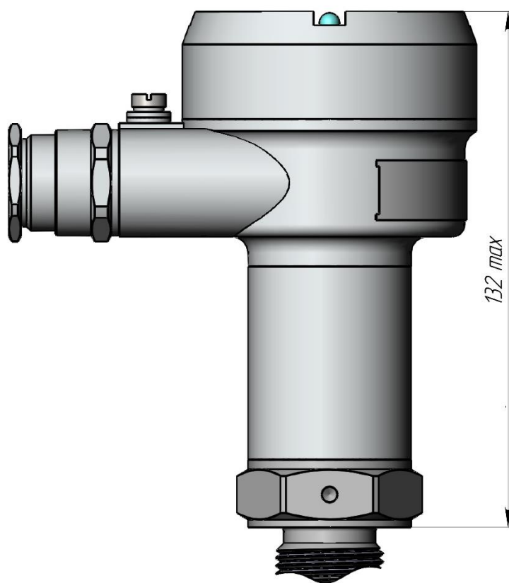
Рисунок В.11 – Габаритные размеры перехода на 160 °С
