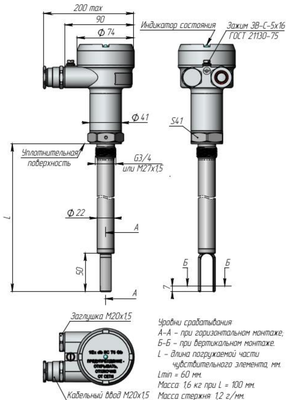
Рисунок В.47 – Габаритные и установочные размеры сигнализатора уровня сыпучих продуктов с вилочным сенсором ВИБРОТЭК-УС-М-В со способом присоединения штуцер G3/4, M27x1,5 с удлиненной вилкой для работы при температурах контролируемой среды не более 160 °С. Для контроля сыпучих материалов небольшой плотности (мука, цемент)
