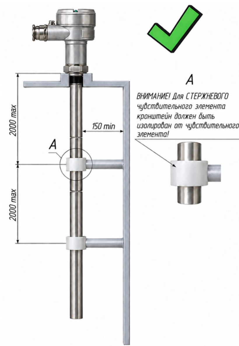
Рисунок 56 – Опоры, необходимые для удлиненного чувствительного элемента
