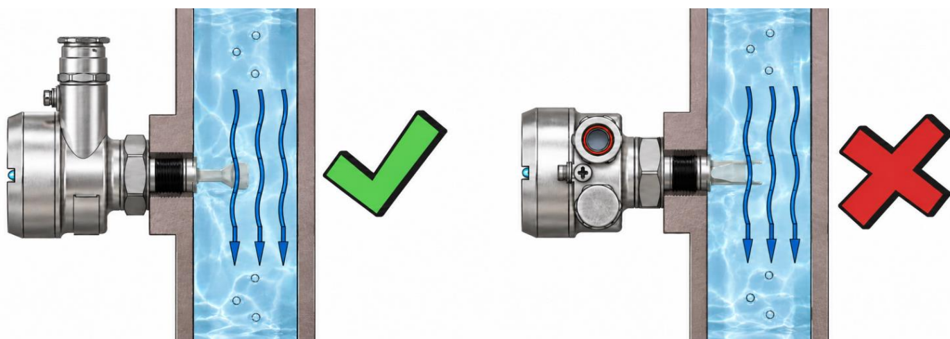
Рисунок 57 – Установка сигнализаторов в трубопроводе
