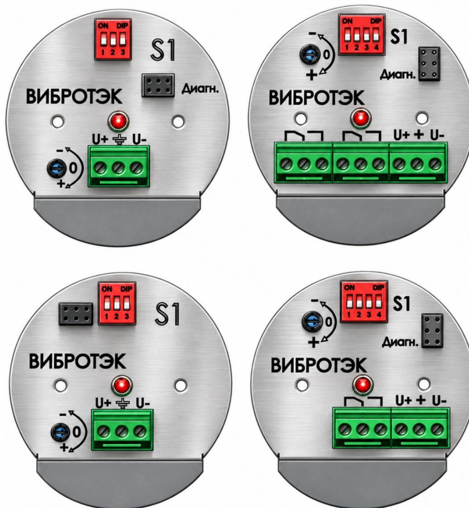
Рисунок 60 – Дискретный регулятор в блоке электронном
