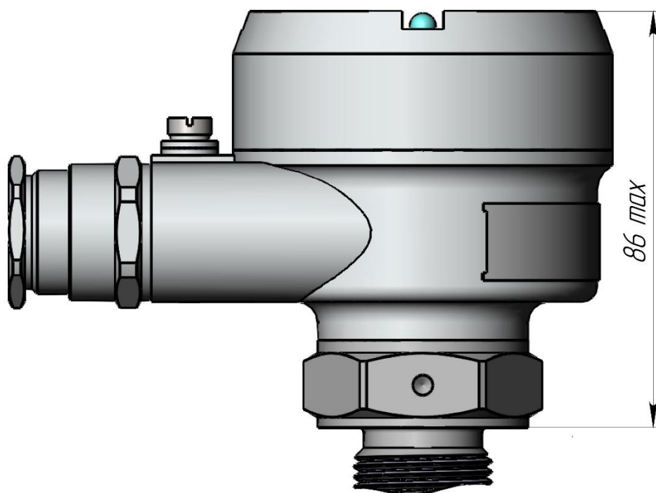
Рисунок В.10 – Габаритные размеры перехода на 100 °С
