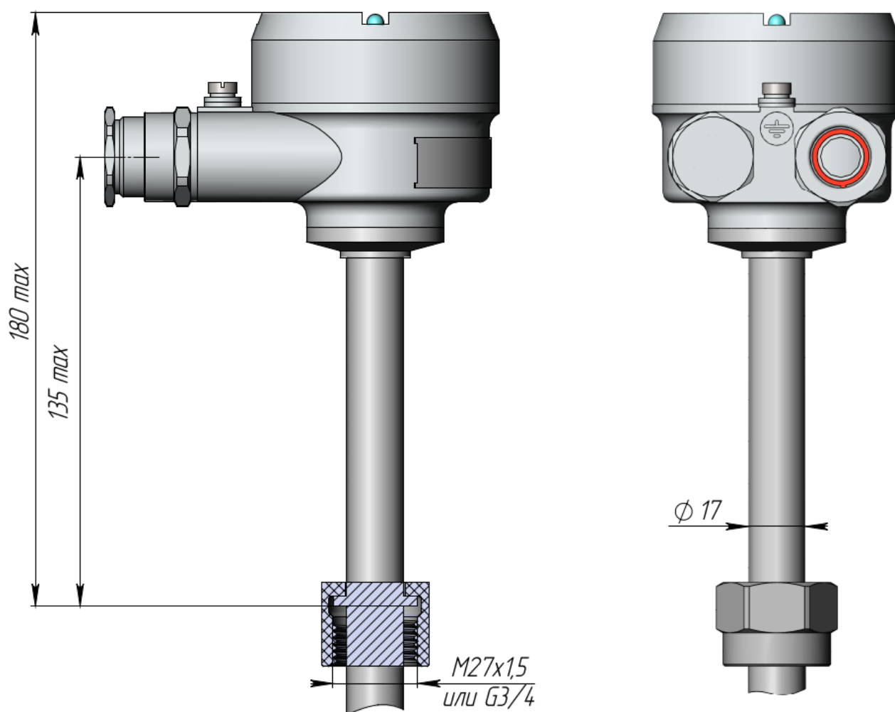
Рисунок В.18 – Габаритные размеры перехода на 160 °С с накидной гайкой
