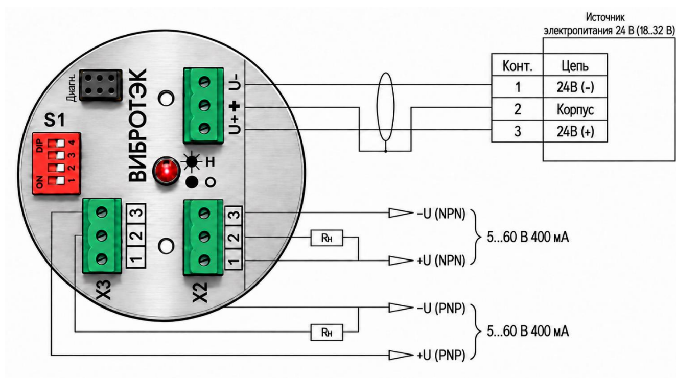
Рисунок 30 – Подключение сигнализатора исполнения TP5
