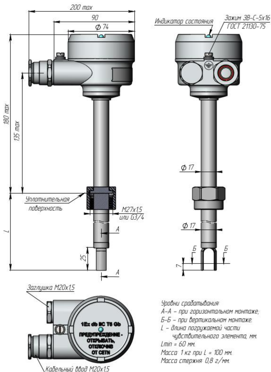
Рисунок В.39 – Габаритные и установочные размеры сигнализатора уровня ВИБРОТЭК-У-М-В со способом присоединения накидная гайка для работы при температурах контролируемой среды не более 160 °С
