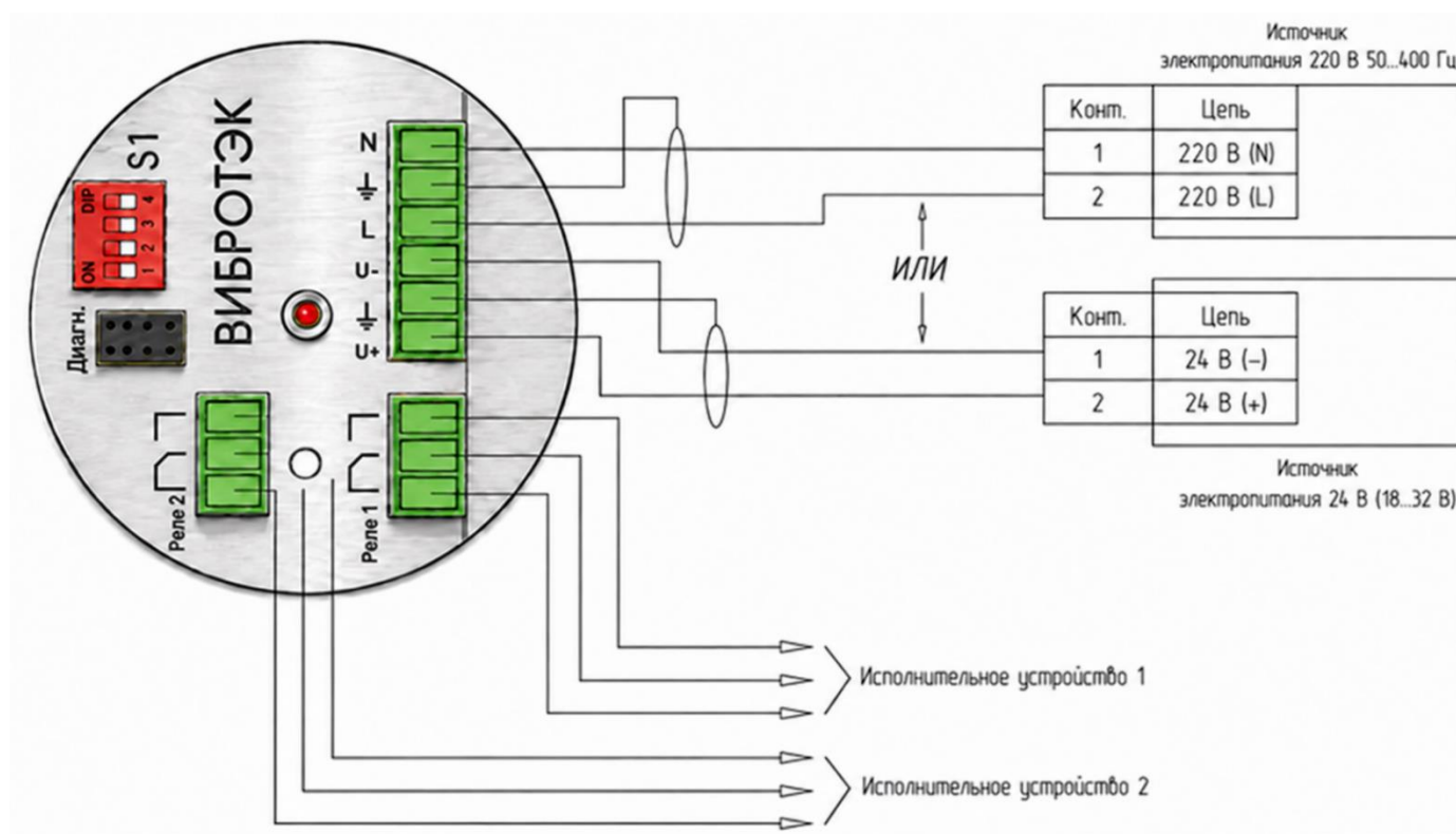
Рисунок 31 – Подключение сигнализатора исполнения Р2, РД, РР (220 В/24 В)
