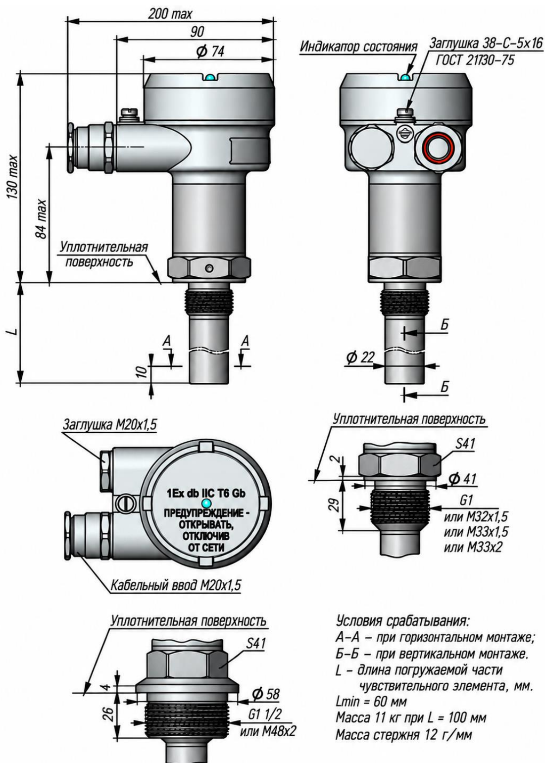
Рисунок В.33 – Габаритные и установочные размеры сигнализатора уровня жидкости стержневого исполнения ВИБРОТЭК-У-М-С со способом присоединения штуцер G3/4 (1; 1 1/2), M27x1,5(2), M32x1,5, M33x1,5(2), M48x2 для работы при температурах контролируемой среды не более 100 °С
