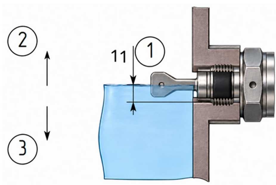
Рисунок 52 – Горизонтальный монтаж
