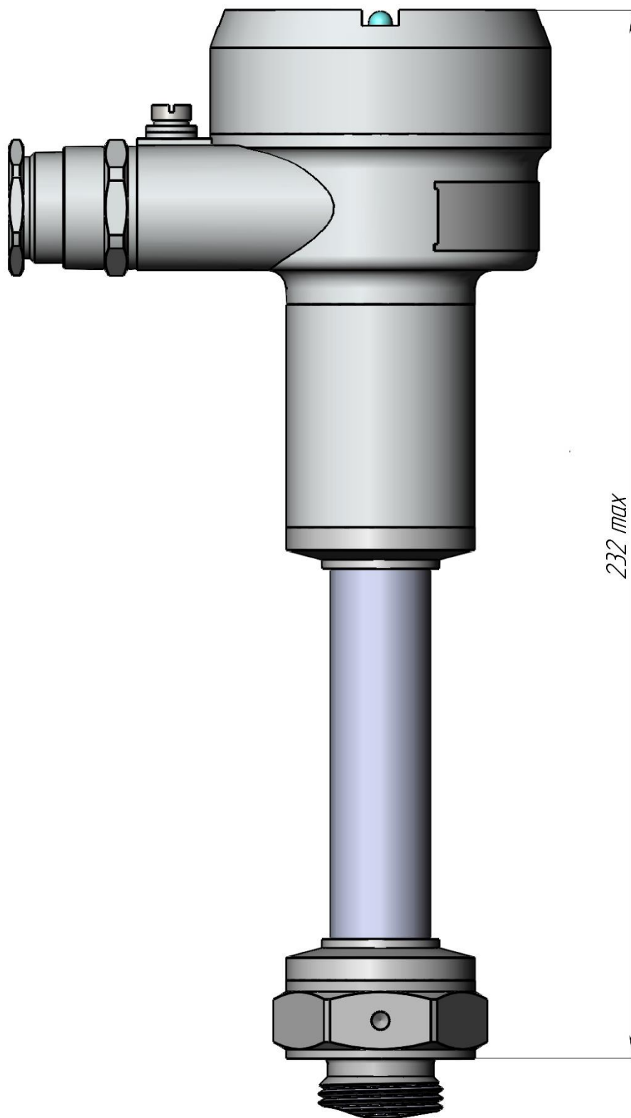
Рисунок В.12 – Габаритные размеры перехода на 250 °С
