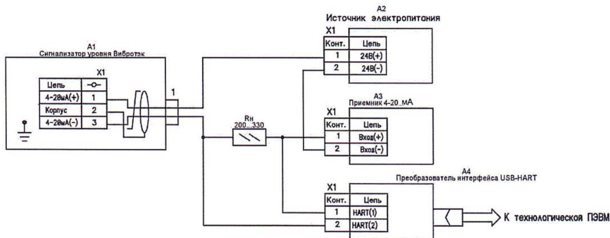
Рисунок Д.2 – Схема электрическая подключения сигнализатора с выходными сигналами A2H, A3H
