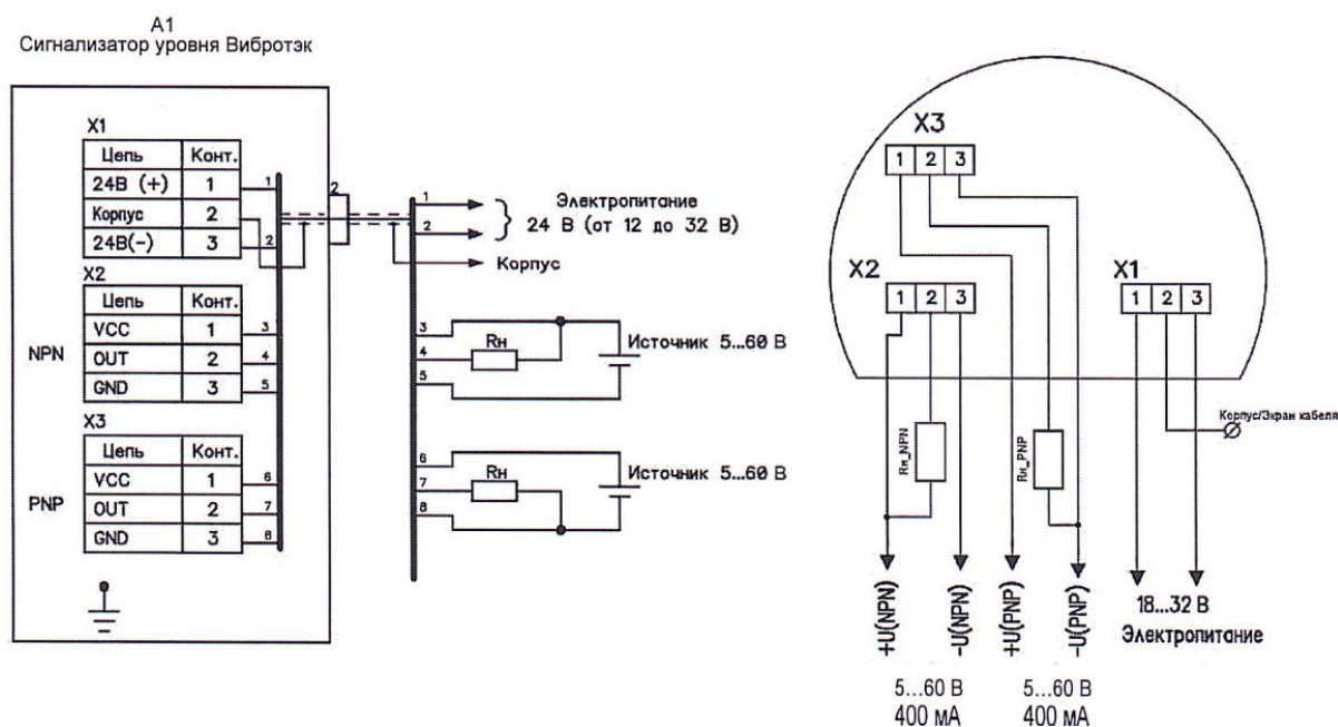
Рисунок Д.6 – Схема электрическая подключения сигнализатора с выходным сигналом TR
