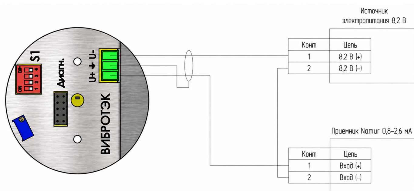
Рисунок 39 – Схема подключения специального исполнения В450 и для сыпучей среды (А1, А2, А3, А4)
