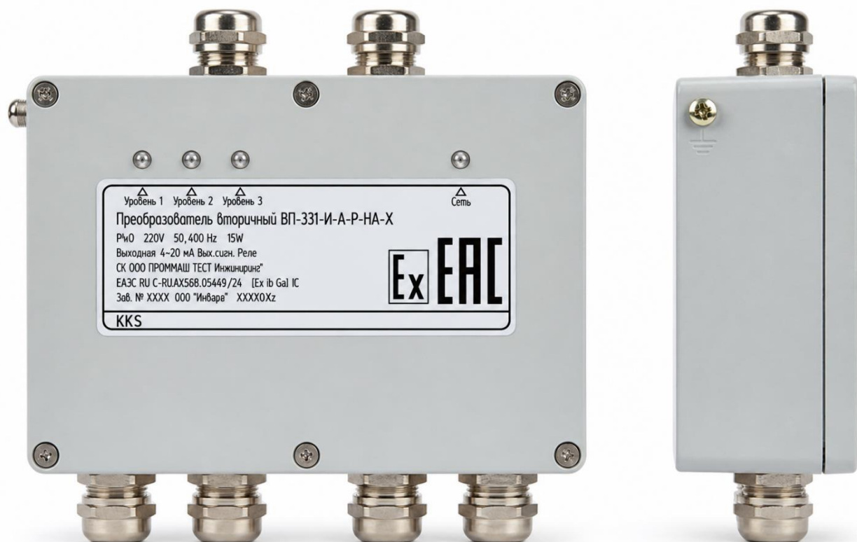
Рисунок 13 – Вторичный преобразователь в алюминиевом корпусе IP66/IP67 для настенного монтажа
