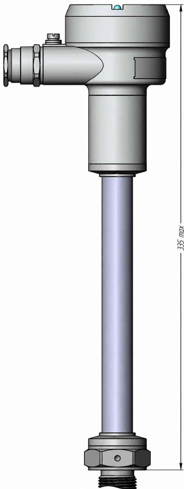
Рисунок В.13 – Габаритные размеры перехода на 450 °С
