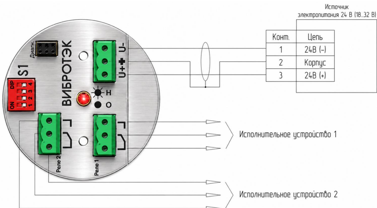
Рисунок 26 – Подключение сигнализатора исполнения P2, РД, РР (24 В)
