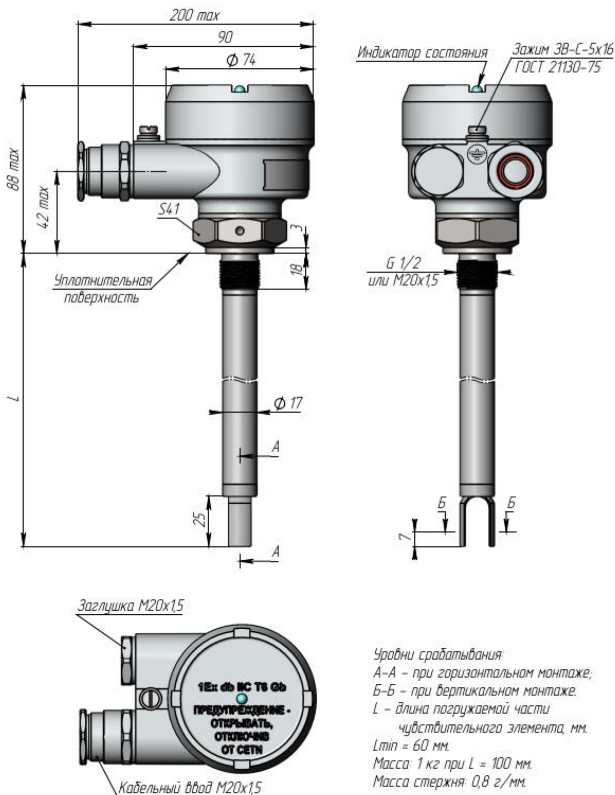
Рисунок В.34 – Габаритные и установочные размеры сигнализатора уровня ВИБРОТЭК-У-М-В со способом присоединения штуцер G1/2, M20x1.5 для работы при температурах контролируемой среды не более 160 °С
