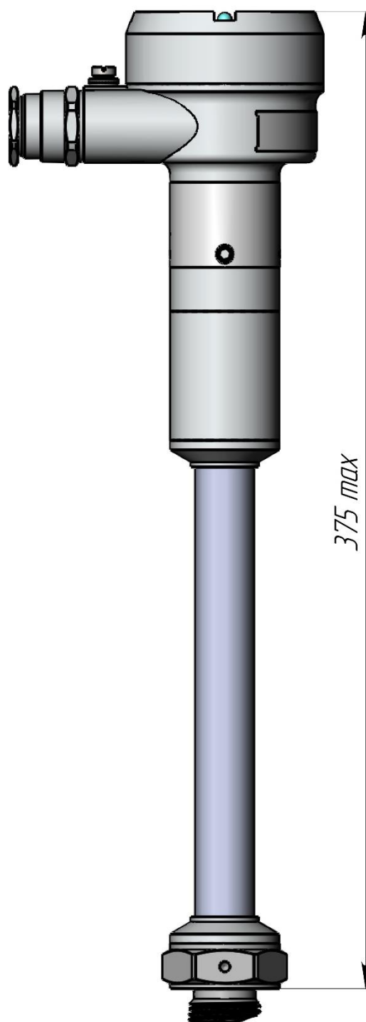
Рисунок В.16 – Габаритные размеры перехода на 450 °С с поворотным механизмом
