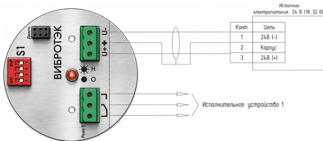
Рисунок 25 – Подключение сигнализатора исполнения P1 (24 В)
