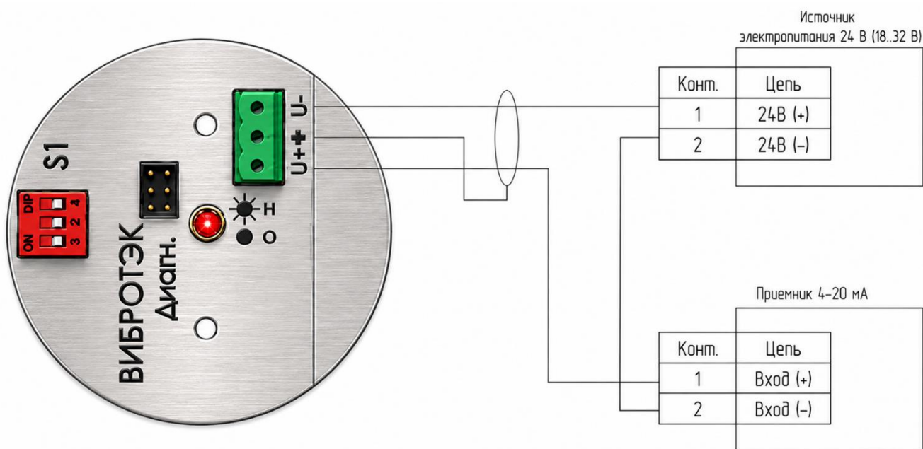
Рисунок 27 – Подключение сигнализатора исполнения А1, А2, А3
