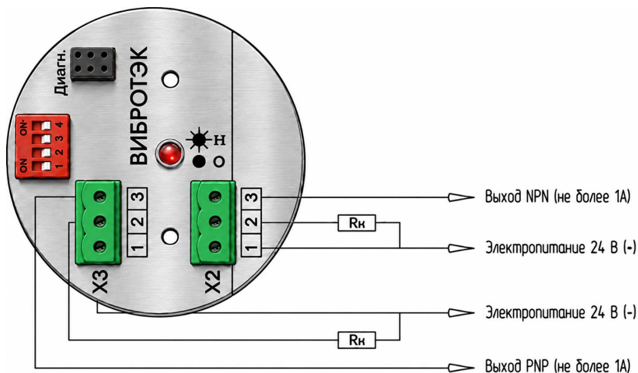
Рисунок 29 – Подключение сигнализатора исполнения TP3
