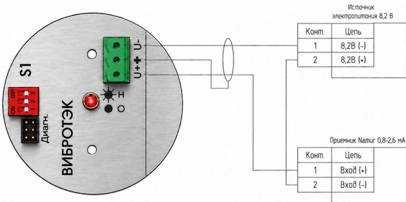
Рисунок 27 – Подключение сигнализатора исполнения А1, А2, А3
