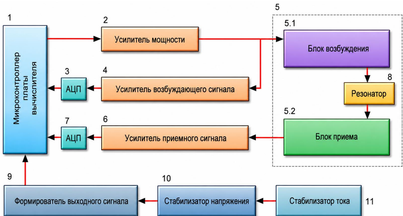
Рисунок 3 – Структурная схема сигнализаторов
