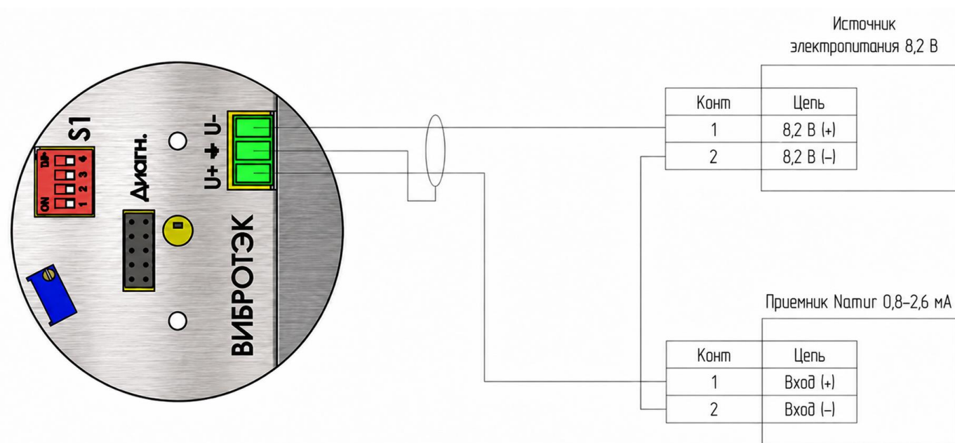
Рисунок 40 – Схема подключения специального исполнения В450 и для сыпучей среды (Natug)
