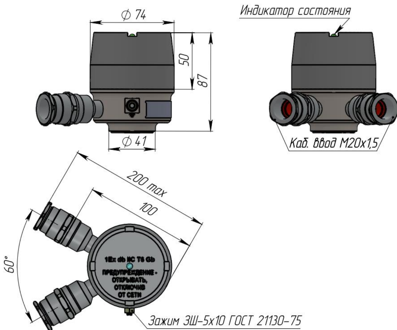
Рисунок В.6 – Габаритные размеры корпуса блока электронного в корпусе из нержавеющей стали для оборудования класса безопасности ЗН (высокая крышка, два кабельных ввода)
