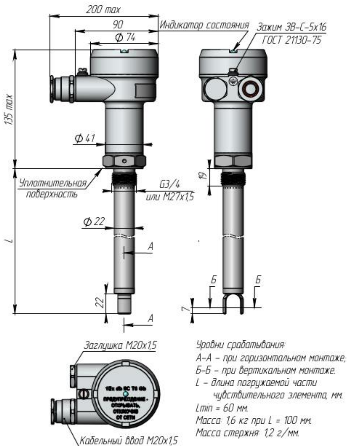
Рисунок В.48 – Габаритные и установочные размеры сигнализатора уровня ВИБРОТЭК-У-М-В со способом присоединения штуцер G3/4, M27x1,5 для работы при температурах контролируемой среды не более 160 °С. Для вязких сред и для контроля твёрдого осадка в жидкости
