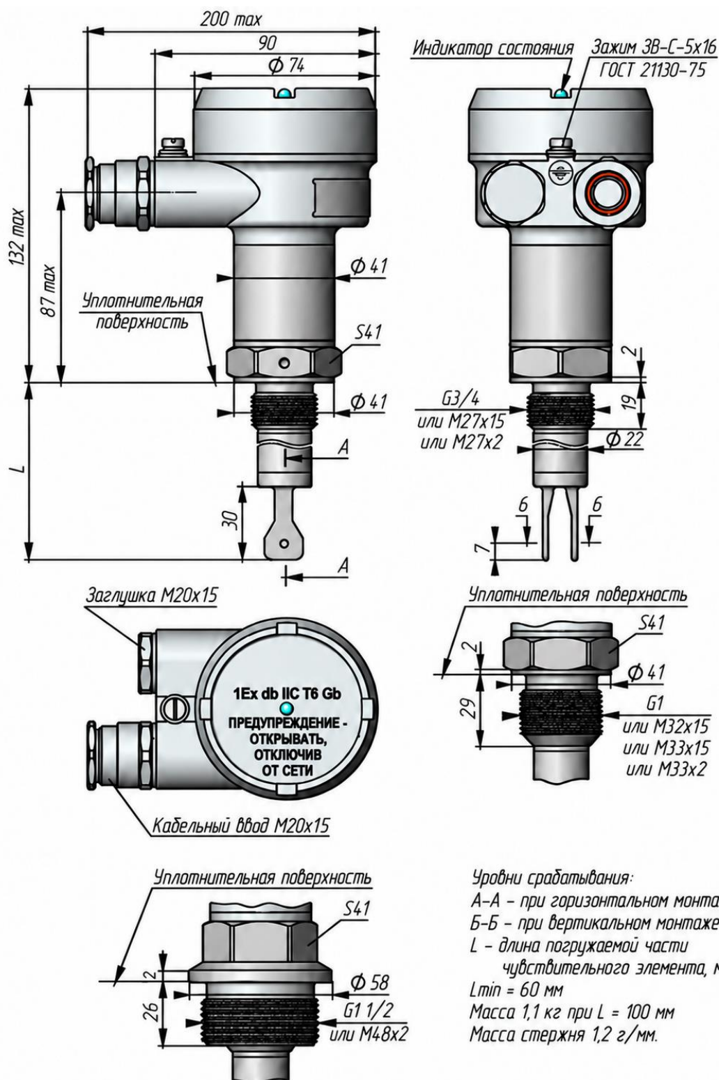
Рисунок В.32 – Габаритные и установочные размеры сигнализаторов уровня жидкости ВИБРОТЭК-У-М-В исполнения В100, В160 и В250 со способом присоединения штуцера G3/4 (1; 1 1/2), M27x1,5(2), M32x1,5, M33x1,5(2), M48x2 для работы при температурах контролируемой среды не более 160 °С
