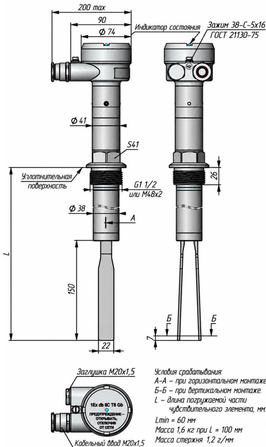
Рисунок В.45 – Габаритные и установочные размеры сигнализатора уровня сыпучих сред с широкой вилкой ВИБРОТЭК-УС-М-В со способом присоединения штуцер G1 1/2, M48x2 с длинной вилкой для работы при температурах контролируемой среды не более 160 °С. Для контроля сыпучих материалов небольшой плотности (мука, цемент)
